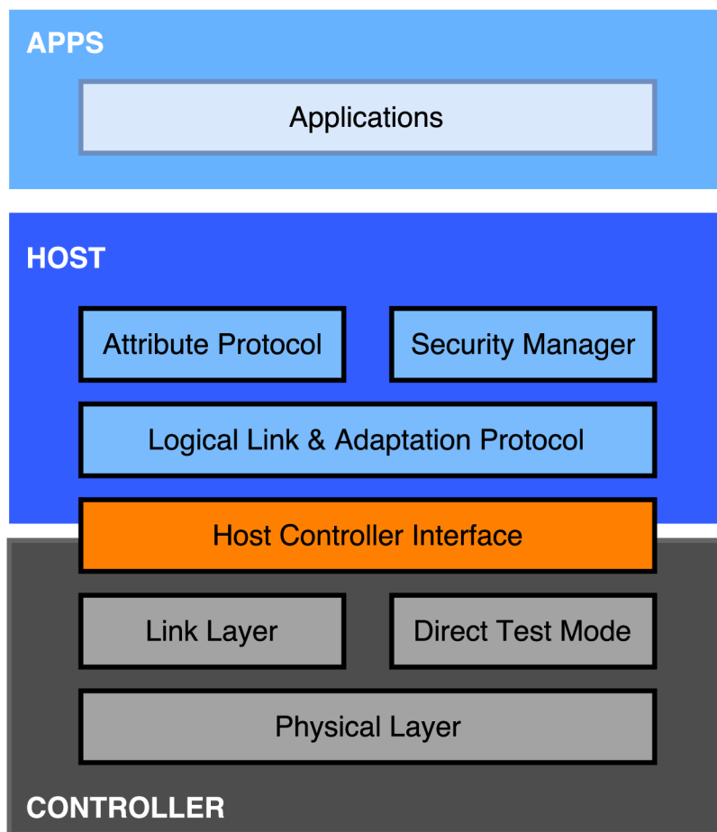
Obrázek 2.1: Bluetooth protocol stack
