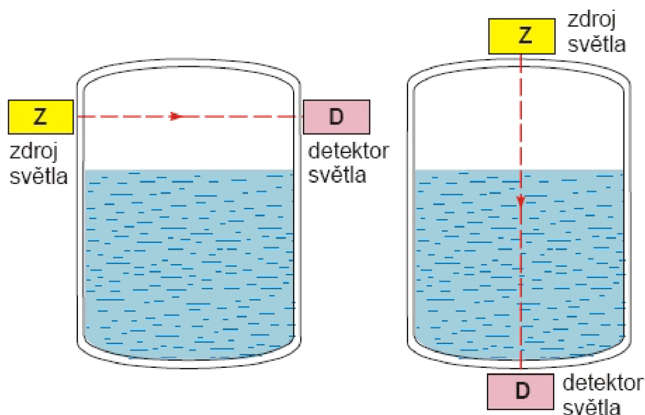
Obr. 15 – Transmisní hladinoměry [11]
