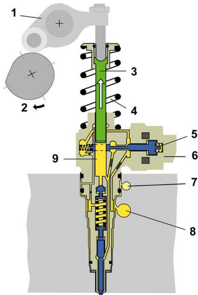
Obrázek 1.6 - Plnění prostoru vysokého tlaku - 1- vahadlo, 2- vstříkovač, 3-píst čerpadla, 4-pružina pístu, 5-jehla ventilu, 6-elektromagnetický ventil, 7-zpětné vedení, 8-přívod paliva, 9-prostor vysokého tlaku (Elektronická učebnice, 2023)
