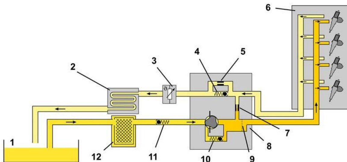
Obrázek 1.1 - Palivová soustava čerpadlo-tryska – 1- nádrž, 2-chladič paliva, 3-snímač teploty paliva, 4-ventil regulace tlaku, 5-bypass, 6-hlava válců, 7-škrťící vrtání, 8-mechanické palivové čerpadlo, 9-sítka, 10-regulační ventil tlaku, 11-zpětný ventil, 12-palivový filtr (Elektronická učebnice, 2023)
