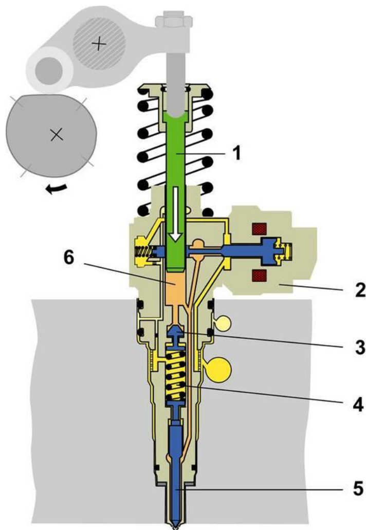
Obrázek 1.8 - Konec pilotního vstříku - 1- píst čerpadla, 2 - elektromagnetický ventil, 3 - kuželový pístkem 4 - pružina, 5 - jehla trysky, 6 -prostor vysokého tlaku (Elektronická učebnice, 2023)
