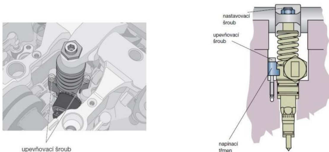
Obrázek 1.10 - Upevnění vstříkovačí jednotky v hlavě válců (Cihlář, 2014)
