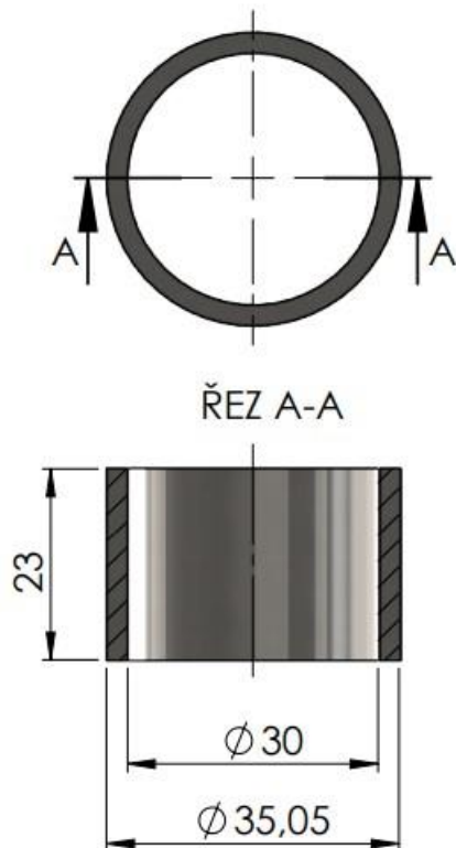
Obrázek 4.11 - Vložka s rozměry
