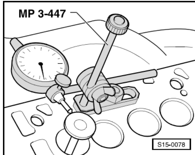
Obrázek 4.15 - Kontrola vodítek ventilů (Firemní literatura, 2004)
