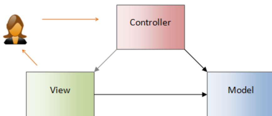
Obr. 25. Vzor MVC [76].
