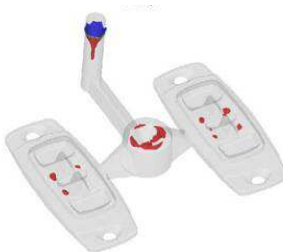
Obr. 11 Na odlitku jsou viditelná místa vzniku bublin [4]
