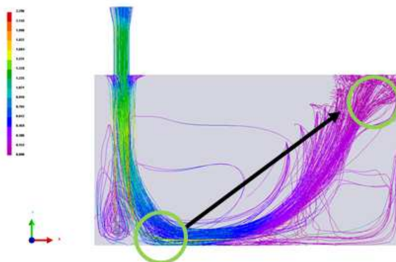
Obr. 7 Místa vyplavení formy [5]
