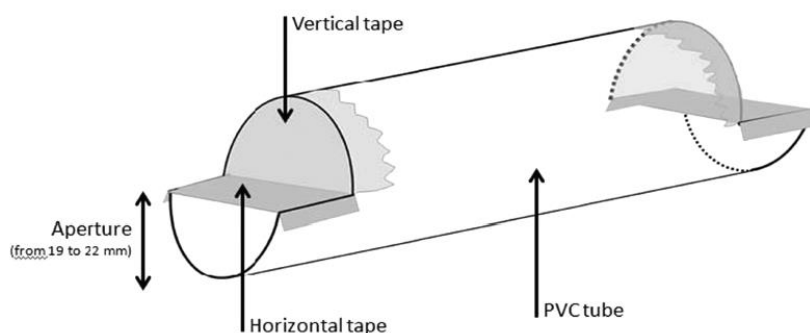
Obr. 18: Schéma chlupové pasti vyrobené za pomoci plastové trubky a oboustranné lepidlo. Nákres převzat ze článku Chiron et al., 2018.
