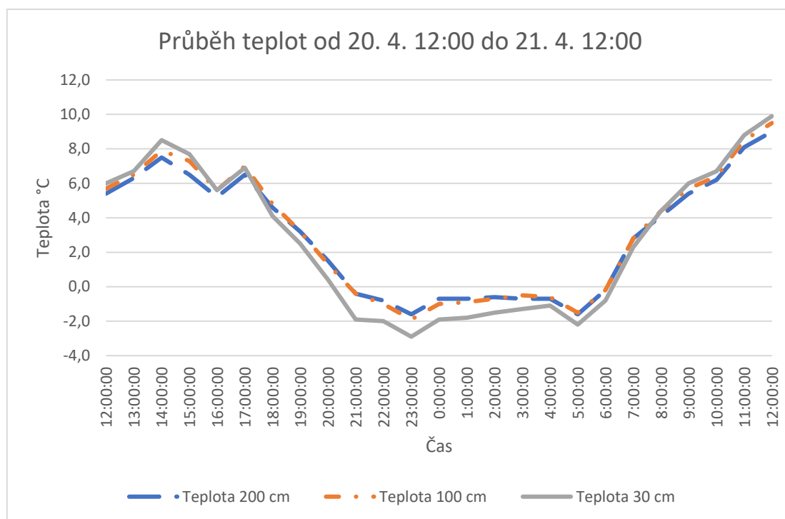
Graf 1: meteorostanice Truba - průběh teplot od 20. 4. 12:00 do 21. 4. 12:00
