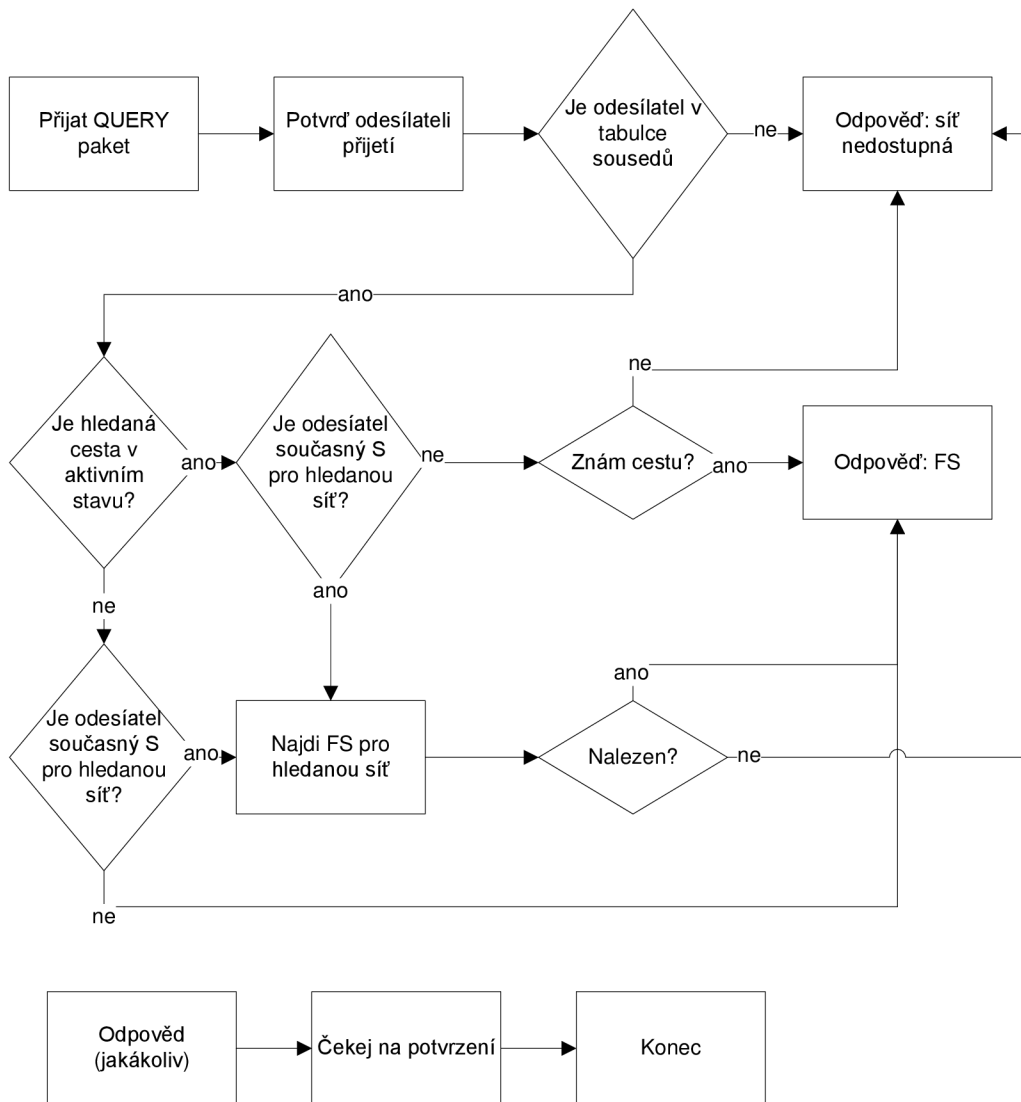
Obrázek 4.7: Proces Přijetí QUERY balíku
