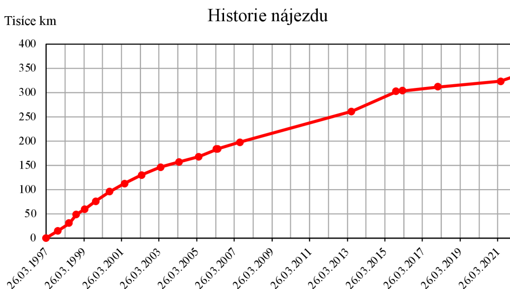
Graf č. 1: Křivka nájezdu vytvořená na základě dostupných dat ze servisních prohlídek a STK
