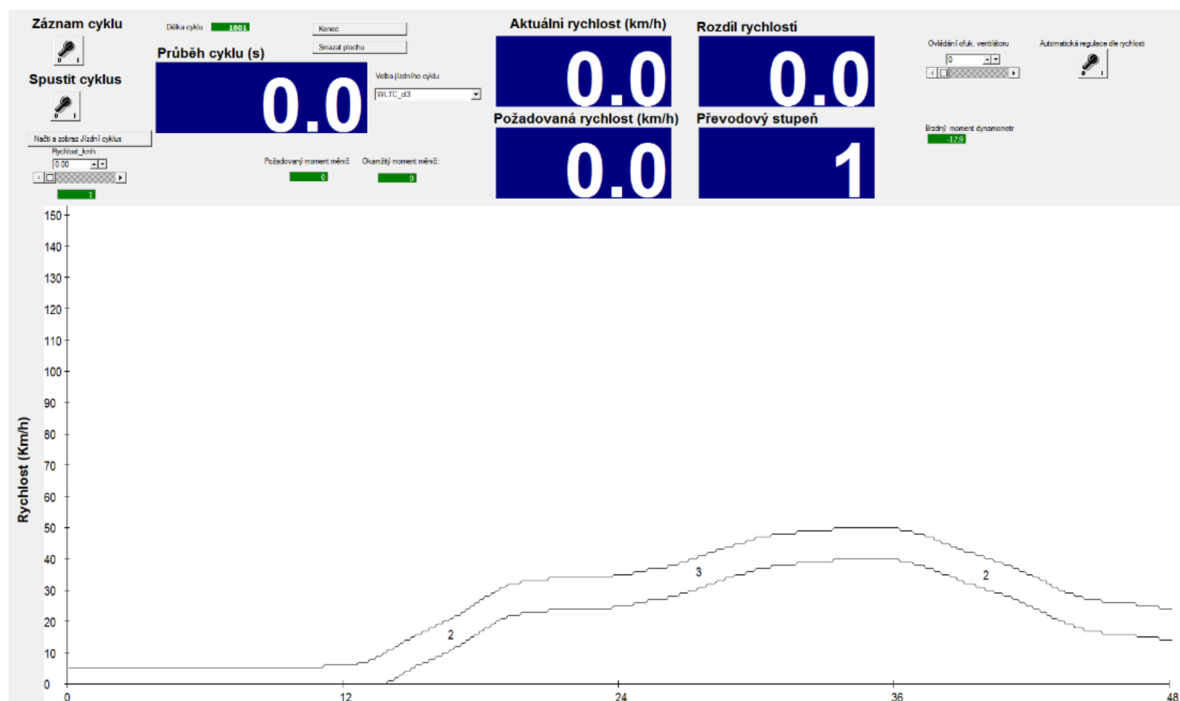
Obrázek č. 18: Příklad mezi rychlosti, ve kterých se musí řidič udržet při zajištění jízdních cyklů v programu ControlWeb. Tuto zrcadlenou obrazovku procesního počítače vidí řidič před sebou na monitoru upevněném na rotačním rameni. Zde je úvodní část cyklu WLTC 3b. [autor]
