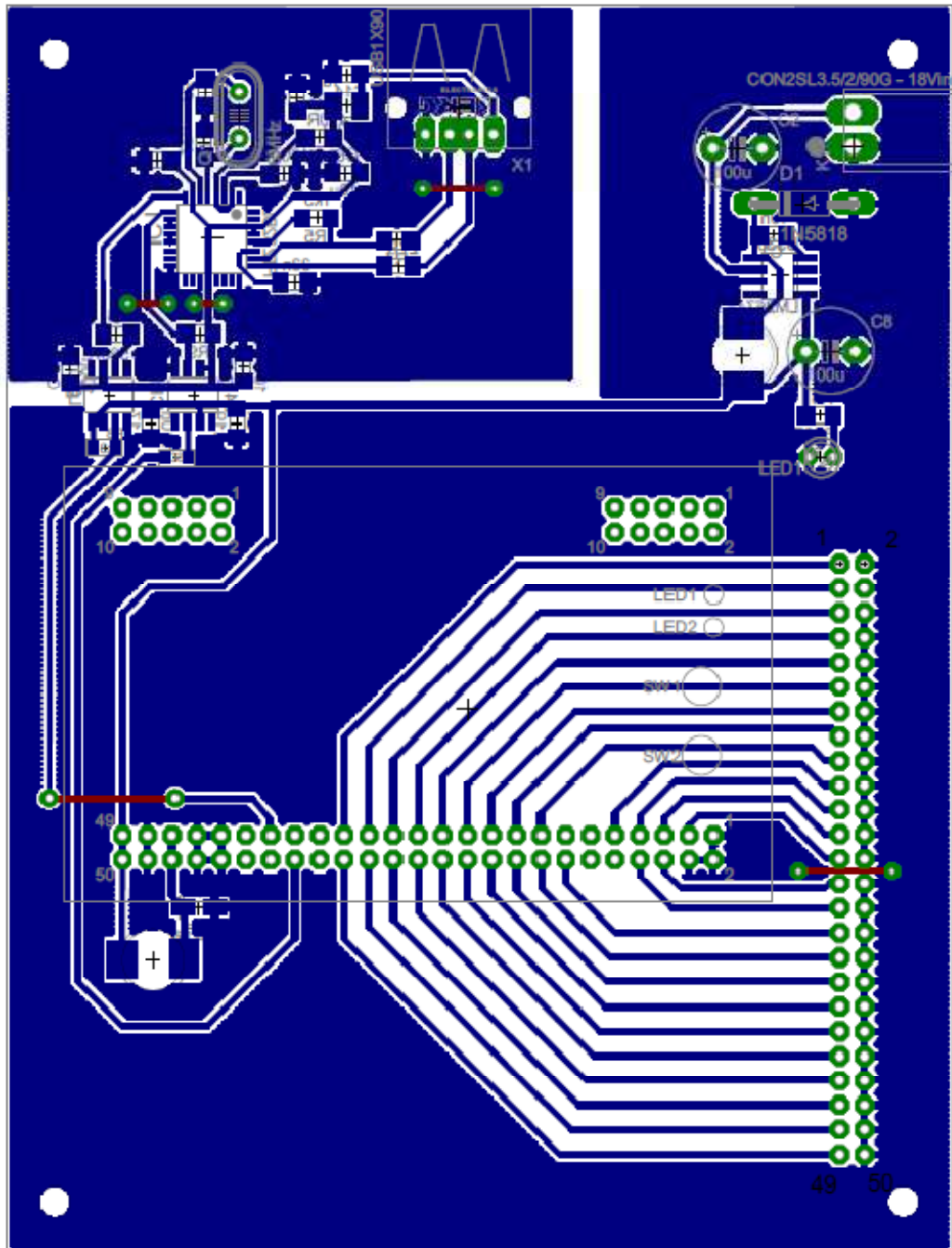
A-10 Návrh desky plošného spoje řídicí a měřicí jednotky
