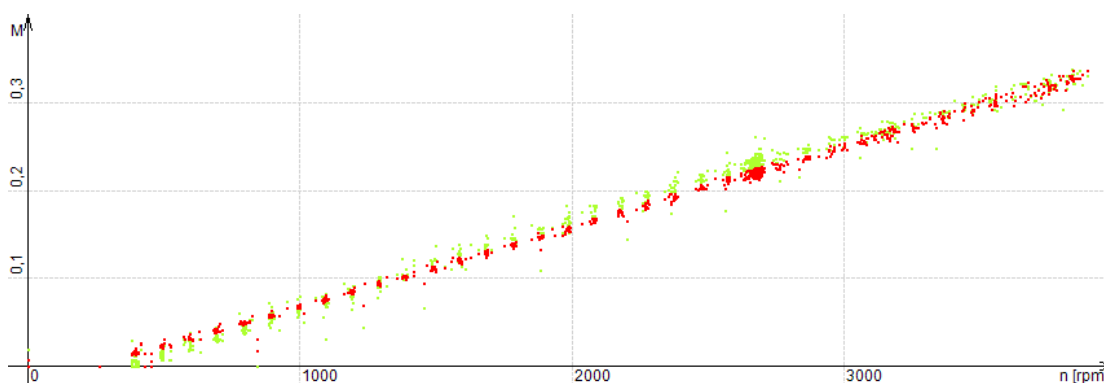
Obr. 8.2 Maximální zatěžovací charakteristika
