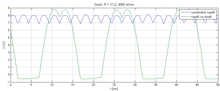
B-6 Porovnání průběhu napětí na tranzistorovém a diodovém usměrňovači při rychlosti 4000 otáček/min. se zátěží 12 \Omega .
