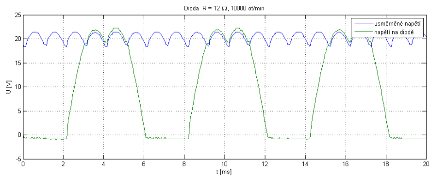
B-9 Porovnání průběhu napětí na tranzistorovém a diodovém usměřovači při rychlosti 10000 otáček/min. se zátěží 12\Omega .
