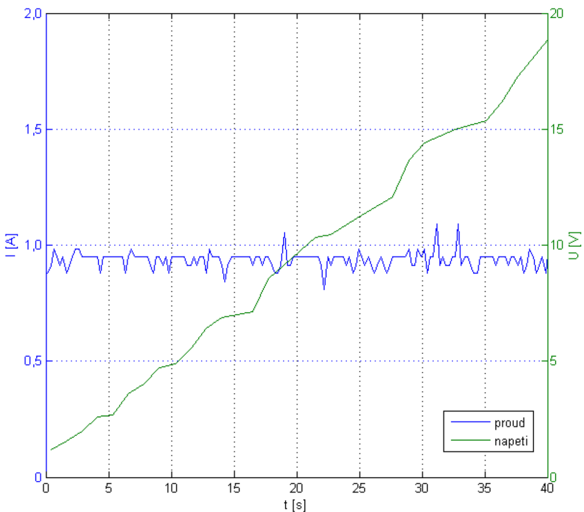
Obr. 5.10 Napětíové zatěžování
