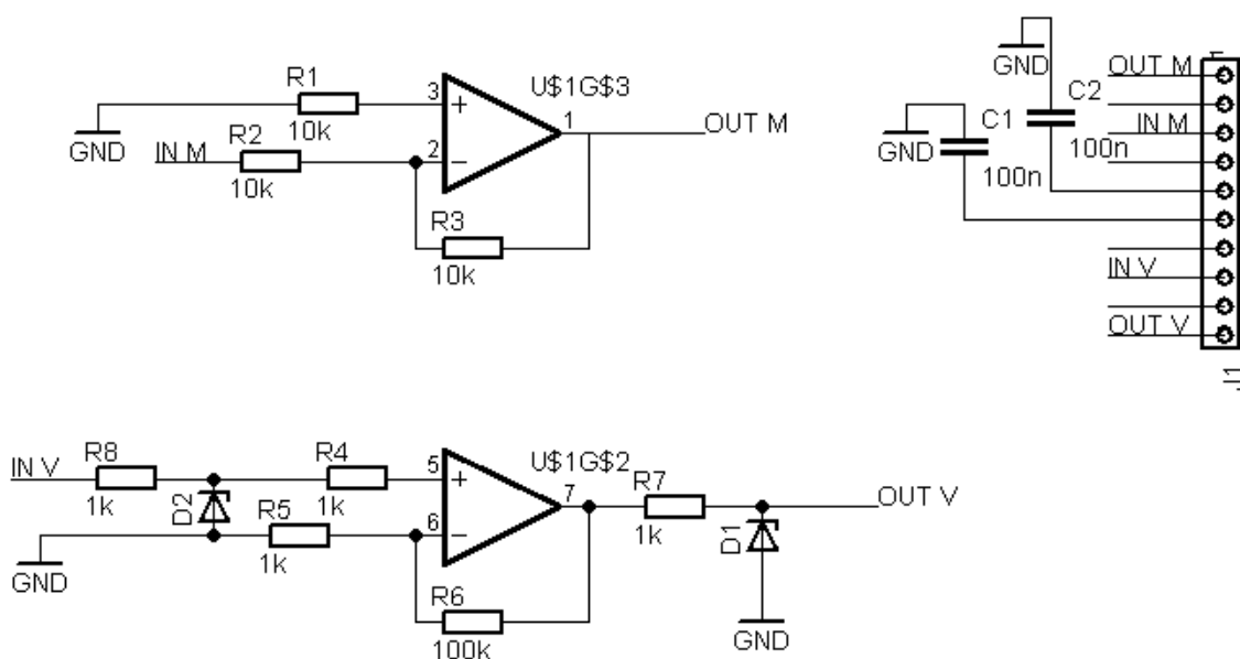
A-12 Schema zapojení napěťového přizpůsobení pro snímač momentu a měření otáček
