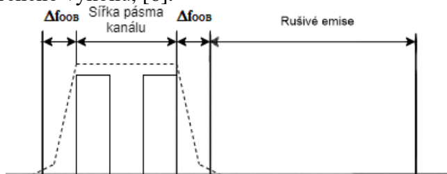
Obr. 2: Zobrazení spektra a jednotlivých oblastí emisí [1]
