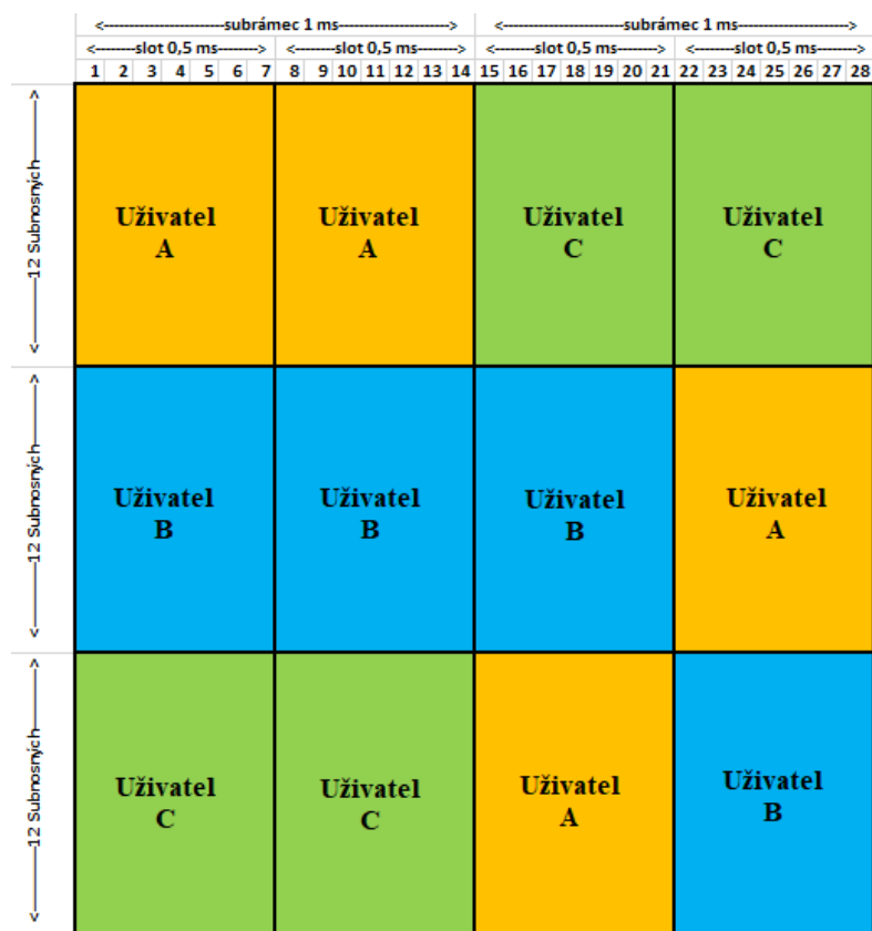
Obr. 2.4: Zobrazení přidělených PRB pro více uživatelů [3]
