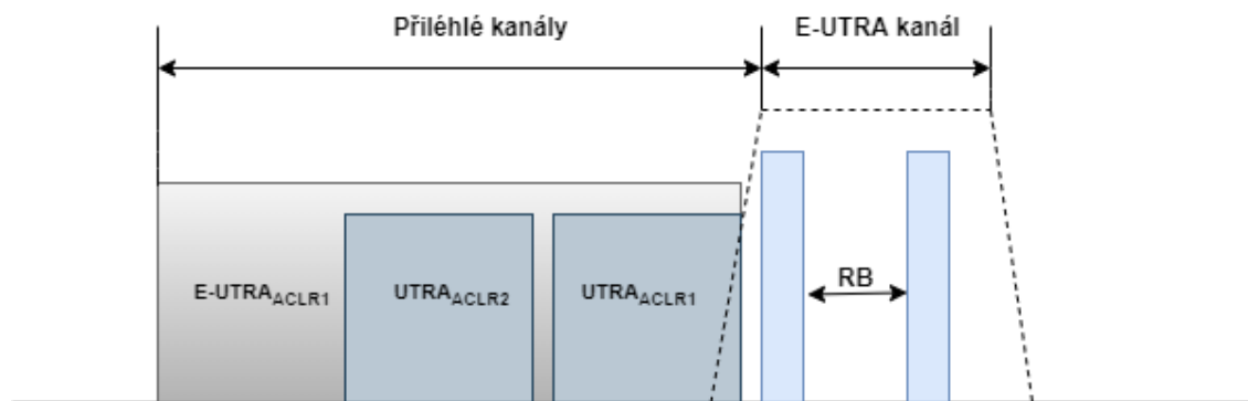
Obr. 3.3: Zobrazení měření ACLR [1]
