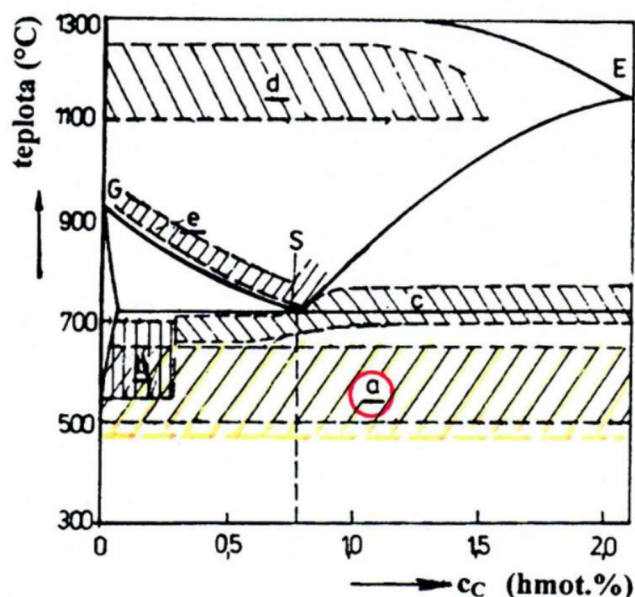
Obr. 2.3 Oblast teplot žíhání na snížení vnitřních pnutí [6]
