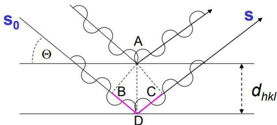
Obr. 2.5 Podmínky difrakce [15]
