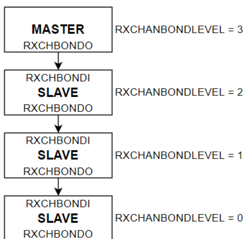
Obr. 2.3 zapojení kanálů při channel bondingu do Daisy Chain [6]
