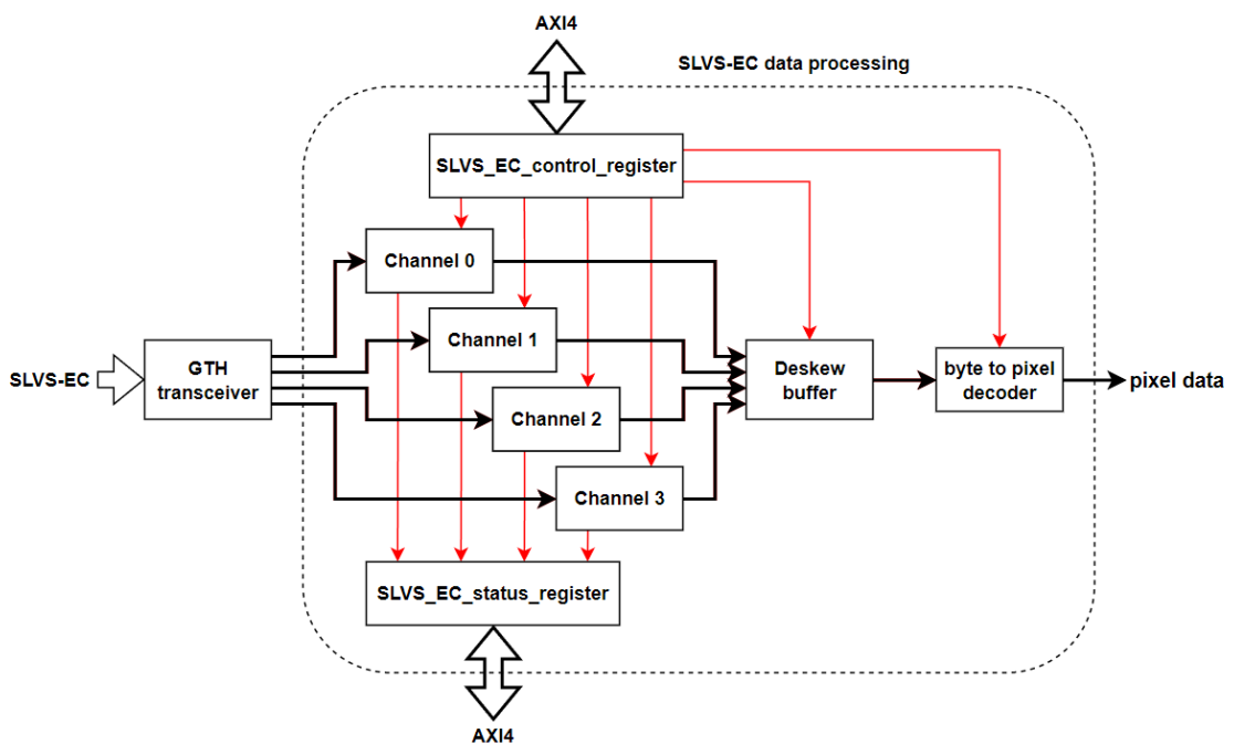
Obr. 2.6 Blokové schéma SLVS-EC data processingu
