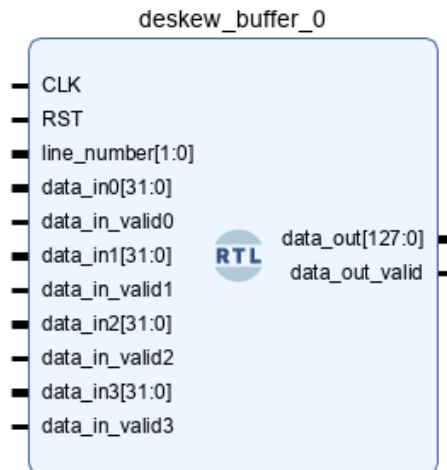
Obr. 2.13 Buffer spojující data z jednotlivých kanálů
