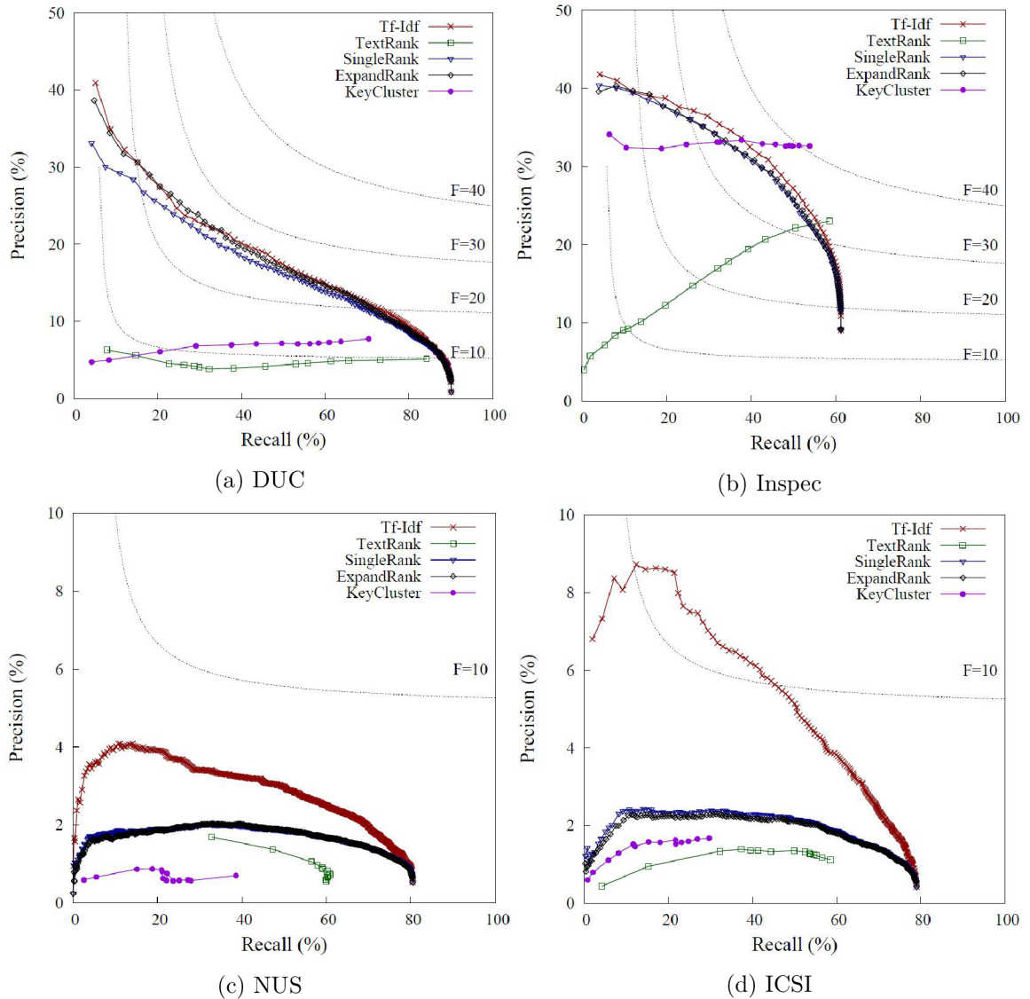
Obr. 6.1: Vzťah medzi hodnotami presnosti a úplnosťou pri rôznych metódach extrakcie, prevzané z [6]
