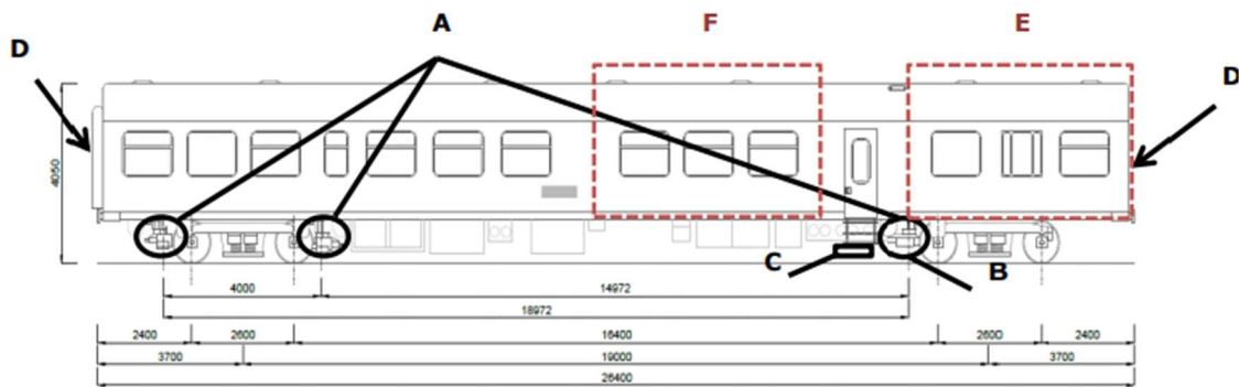
Obr. 3: Schéma MVŽSv [4]
