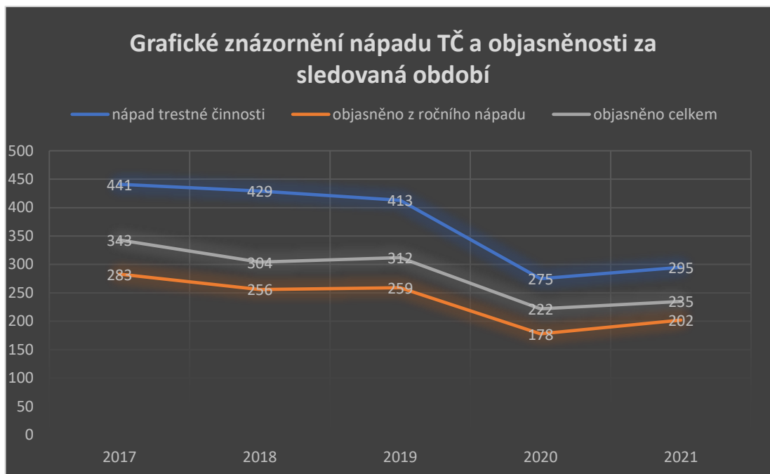
4 - graf nápadu trestné činnosti a objasněnosti
