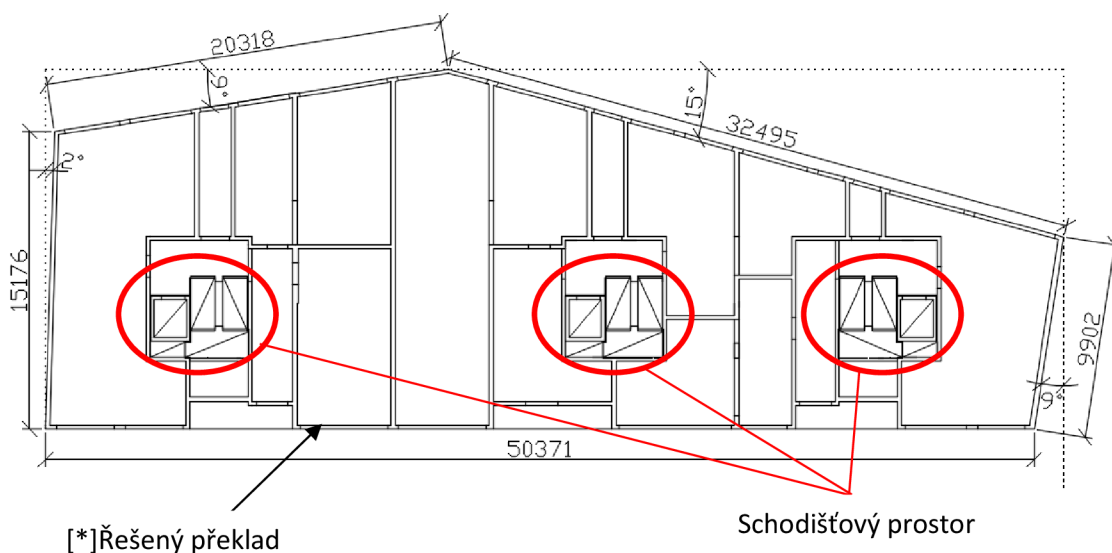
Obrázek 2.1.2: Obrázek půdorysný pohled
