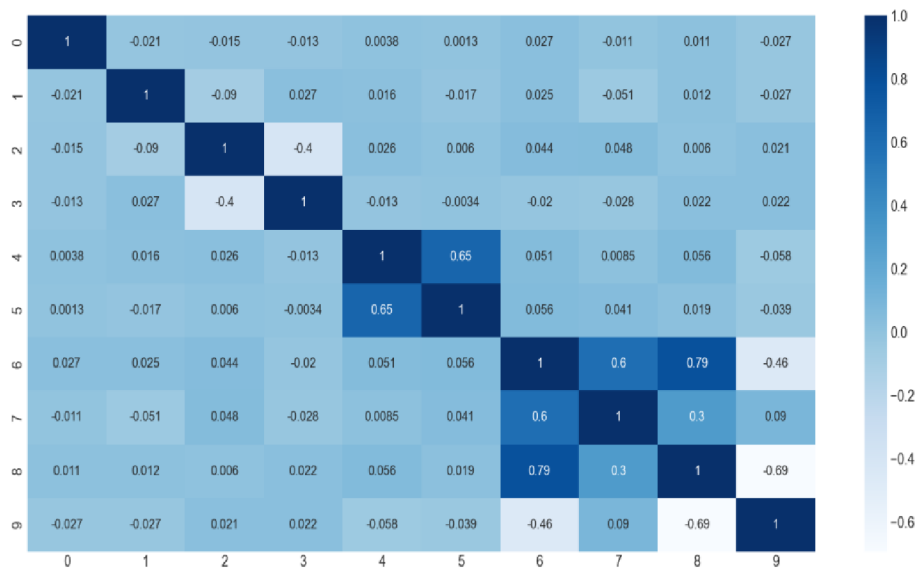
Obrázek 9 - Vizualizace korelační matice daného souboru dat (vlastní zpracování)
