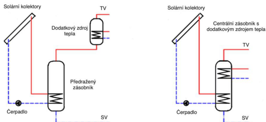
Obr. 2.4 Schéma solární přípravy teplé vody: vlevo – s předehřívacím zásobníkem, vpravo – s bivalentním zásobníkem [24]
