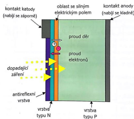
Obr. 2.8 Vznik fotovoltaického napětí na struktuře s přechodem PN [33]
