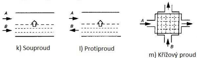
Obr. 1-1 Dělení výměníků [2].
