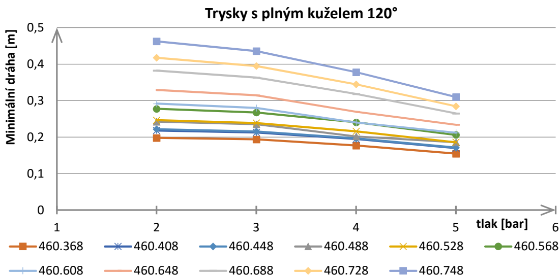
Obr. 5-9 Graf závislosti požadované dráhy na tlaku pro trysky s plným kuzelem 120°.
