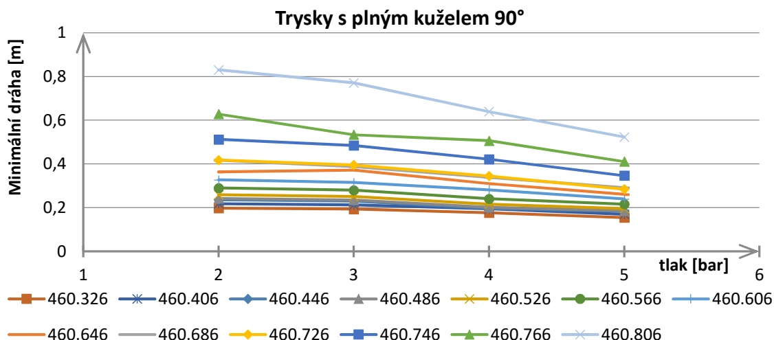
Obr. 5-8 Graf závislosti požadované dráhy na tlaku pro trysky s plným kuzelem 90°.
