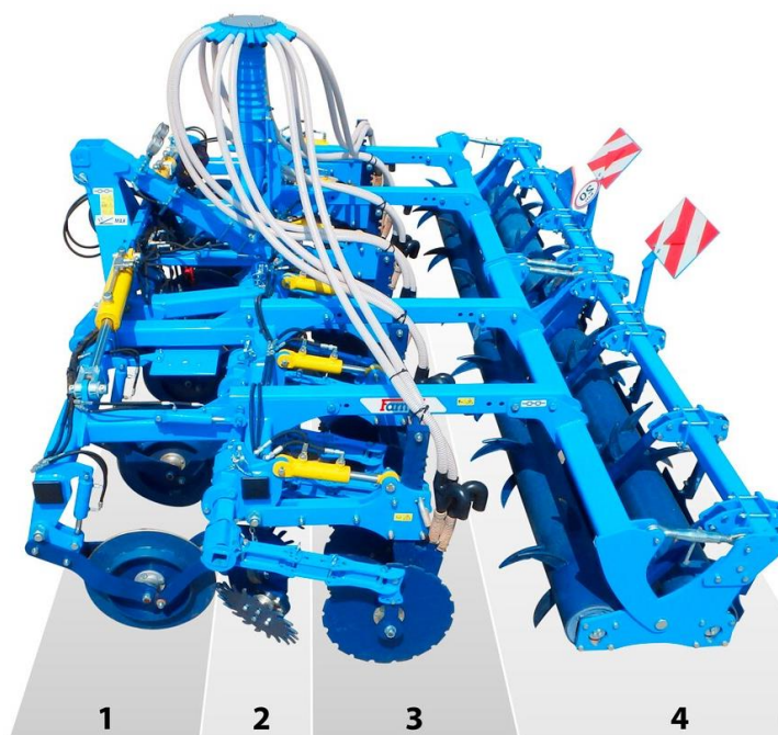
Obrázek 1 Pásový kypřič Farmet STRIP-TILL (farmet.cz)
