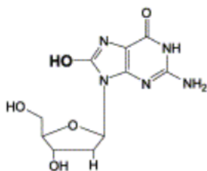
Obrázek 5 - Strukturní vzorec 8-hydroxy-2'-deoxyguanosinu (upraveno podle Wu 2004).
