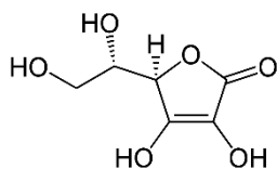
Obrázek 8 - Vzorec kyseliny L-askorbové. (Upraveno podle Oroian & Escriche 2015)
