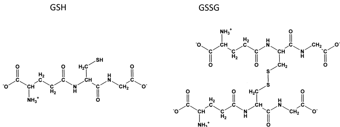
Obrázek 6 - Strukturní vzorce redukovaného glutathionu GSH a oxidovaného GSSG. (Upraveno podle Krezel & Bal 2004).
