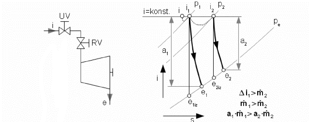
Obrázek 9 Regulace škrcením [8]
