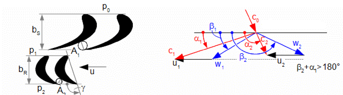
Obrázek 2 Rozvinutý válcový řez akčního stupně a jeho rychlostní trojúhelník [3]
