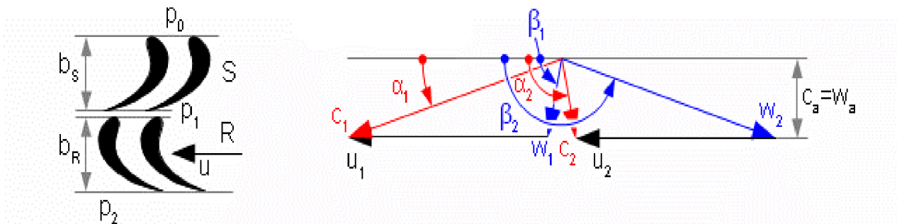
Obrázek 3 Rozvinutý válcový řez reakčního stupně a rychlostní trojúhelník; \rho = 0,5 [3]
