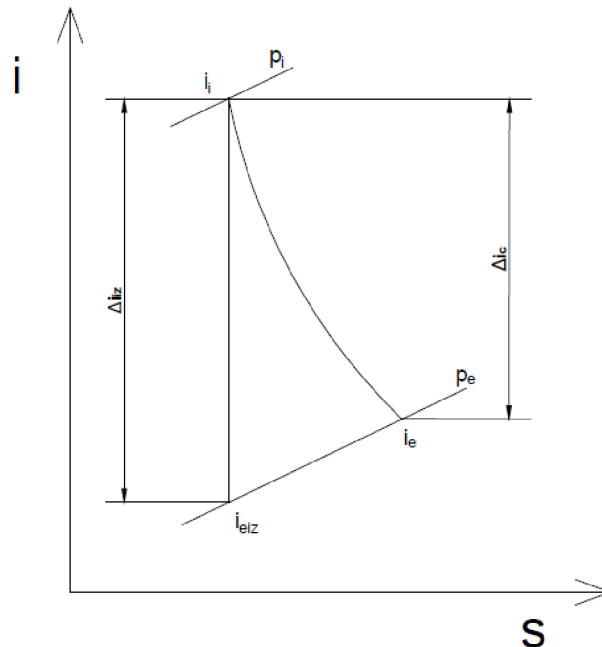
Obrázek 21 i-s diagram expanze páry v parní turbíně
