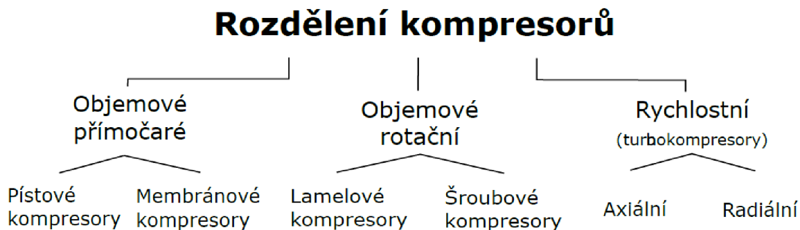
Obrázek 13 Rozdělení kompresorů
