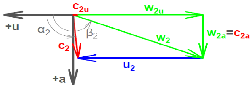
Obrázek 25 Rychlostní trojúhelník výstupních rychlostí z rotoru
