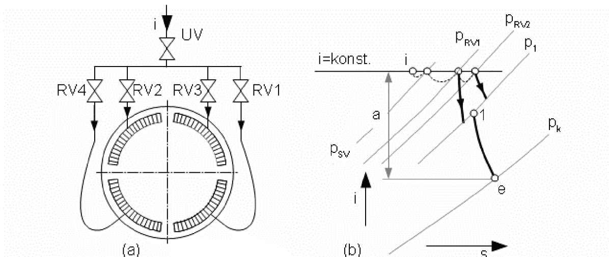
Obrázek 10 Skupinová regulace výkonu [8]
