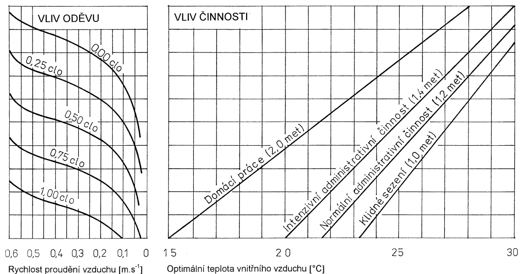
Obr. 14 Vztahy mezi rychlostí proudění vzduchu, oděvem, činnostmi a optimální vnitřní teplotou 1,00 \text{ clo} = 0,16 \text{ m}^2 \cdot \text{K} \cdot \text{W}^{-1} , 1 \text{ met} = 58 \text{ W} \cdot \text{m}^{-2} , \varphi_{ai} = 50 \%
