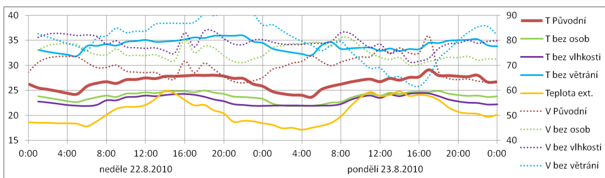
Obr. 56 Začátek pracovních dnů – průběhy teploty vzduchu a relativní vlhkosti při různých okrajových podmínkách v obývacím pokoji ve dnech 22.8-23.8. 2010
