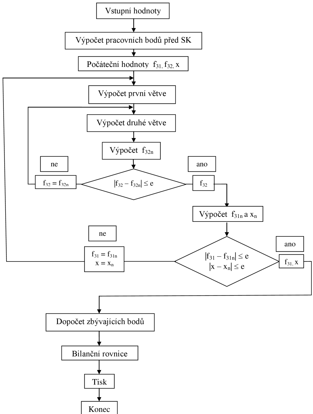
Obr. 17 Schéma postupu výpočtu pro paralelní řazení turbin
