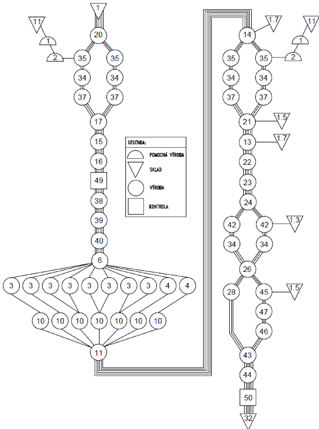
Obr. 28: Schéma materiálového toku pro výrobu vícevrstvých DPS
