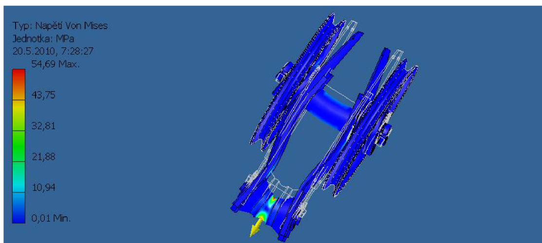
Obr. 3.3: Maximální napětí
