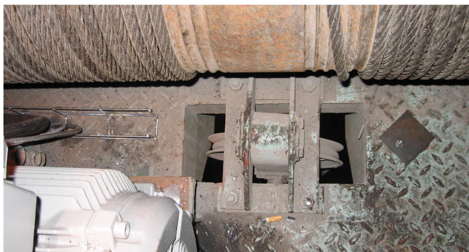
Obr. 2.8: Původní konstrukce vyrovnávací kladky
