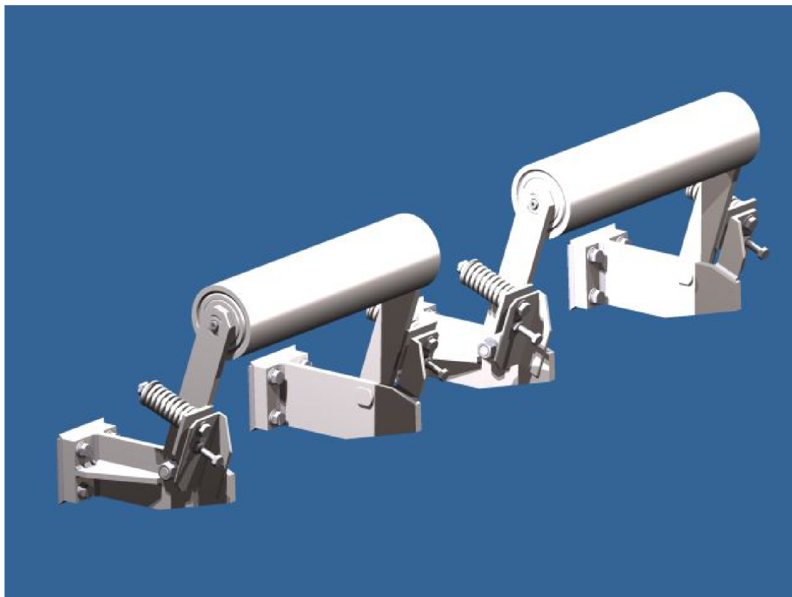
Obr. 3.7: Návrh přitlačování lan
