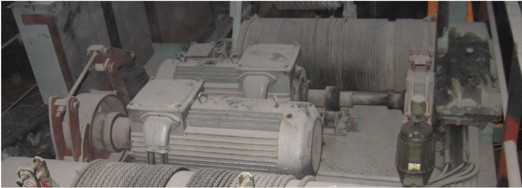
Obr. 2.3: Původní pohony hlavního a pomocného zdvihu
