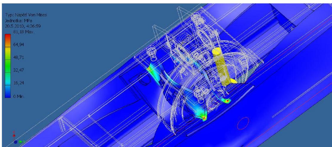
Obr. 3.10: Maximální napětí
