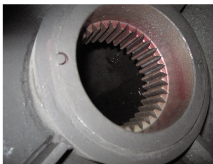
Obr. 3.6: Detail náboje
