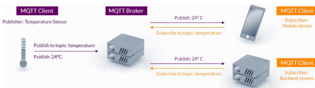
Obrázek 3.5 Architektura MQTT[19]
