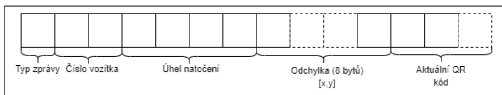
Obrázek 3.12 Struktura paketu typu zprávy 0x02
