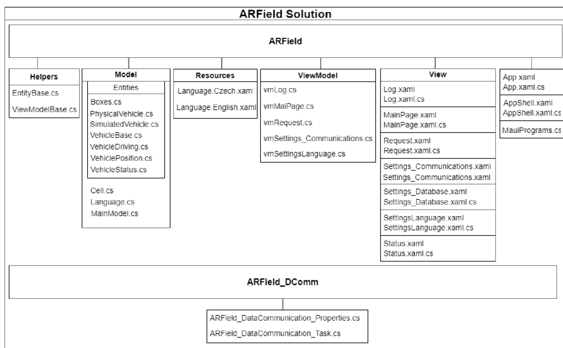
Obrázek 5.1 Struktura projektu
