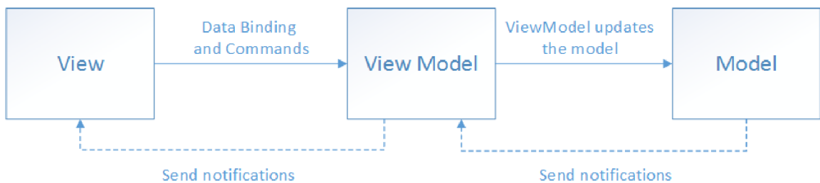
Obrázek 4.2 Struktura MVVM [30]
