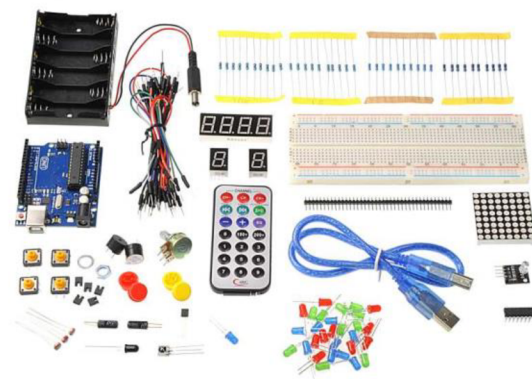
Obrázek 31: Základní modul stavebnice Arduino [45].
