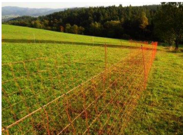
Obrázek 12 Zdvojená přenosná vodivá síť, Zdroj AOPK ČR, 2023
