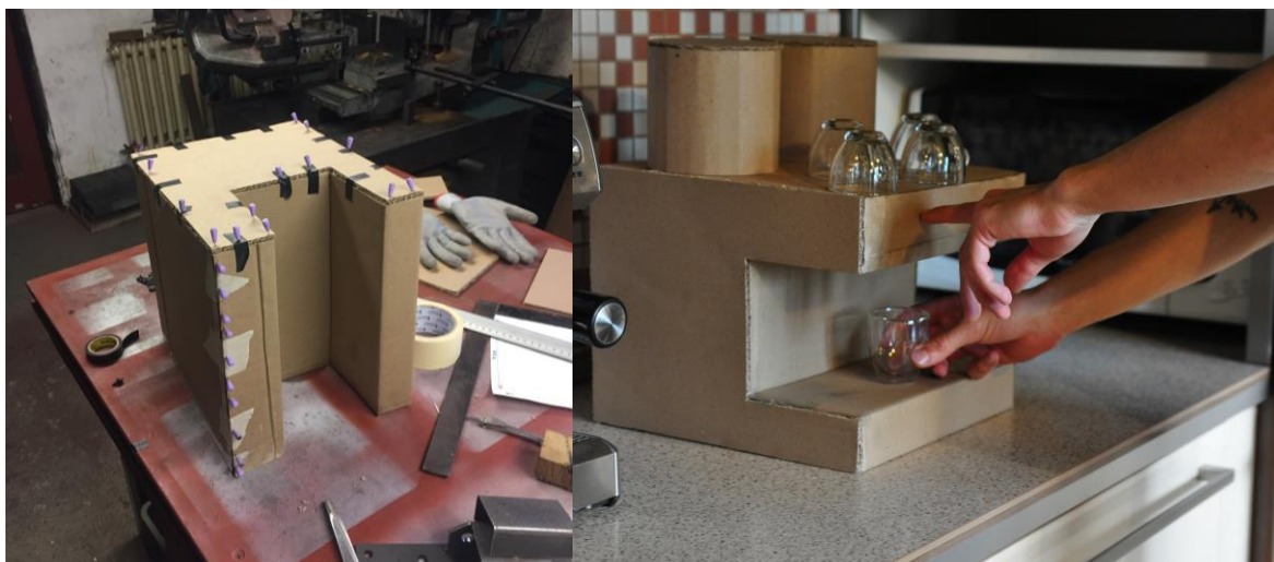
Obr. 6-6 Ergonomický model
