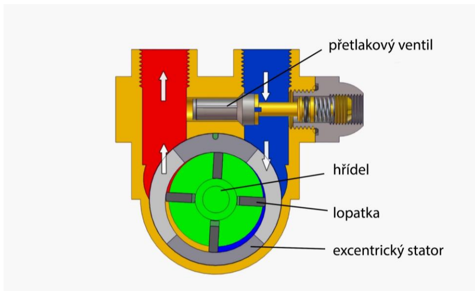
Obr. 2-13 Rotační čerpadlo - řez
