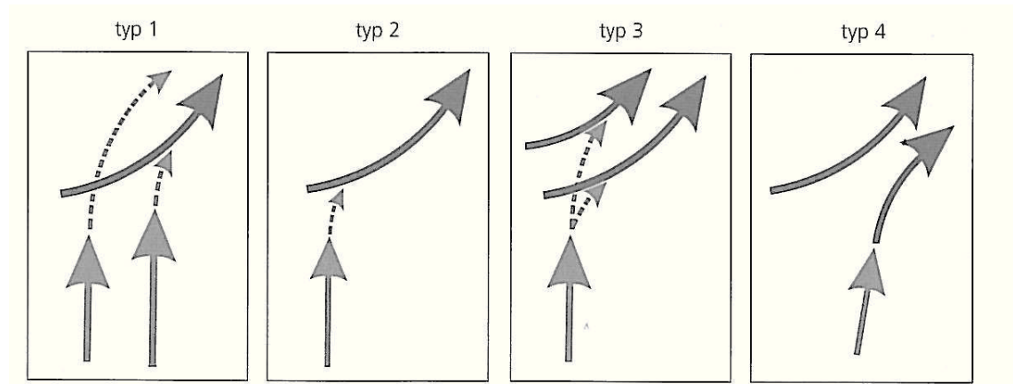
Obr. 1.12 Typy uspořádání vjezdu do turbo-okružní křižovatky
