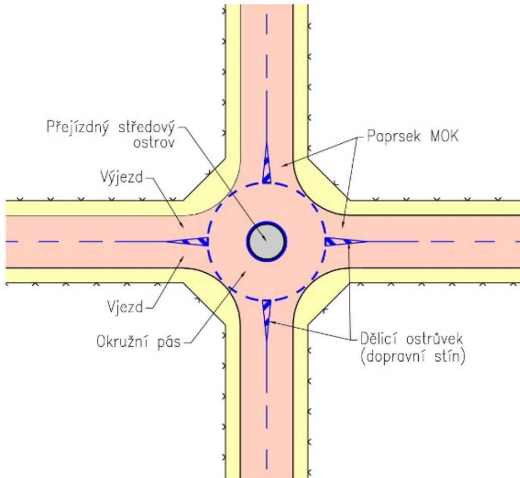
Obr. 1.3 Schéma miniokružní křižovatky
