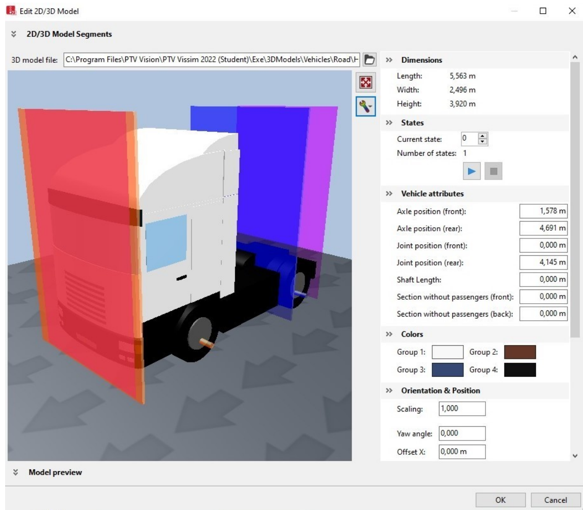
Obr. 2.8 Editace vozidla
