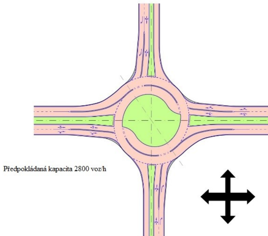
Obr. 1.7 Schéma základní TOK (šipky znázorňují rozložení intenzit dopravy)
