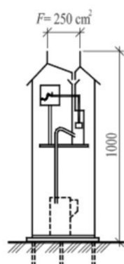
Obr. 3: Ombrograf (Starý, 2005)
