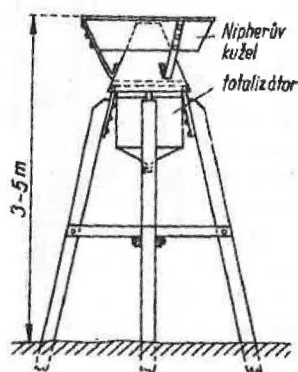
Obr. 2: Totalizátor (Kemel, 1996)
