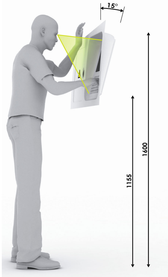
7.11 Umiestnenie hlavného riadiaceho panelu
