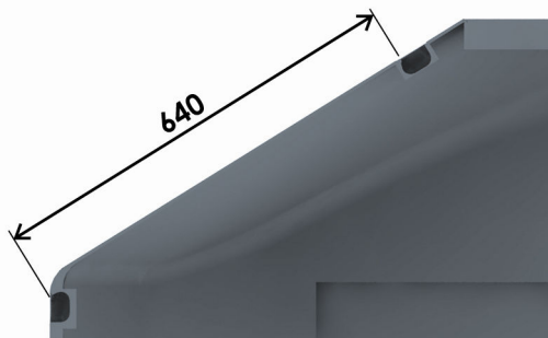
7.5 Profil zapustených držiadiel
