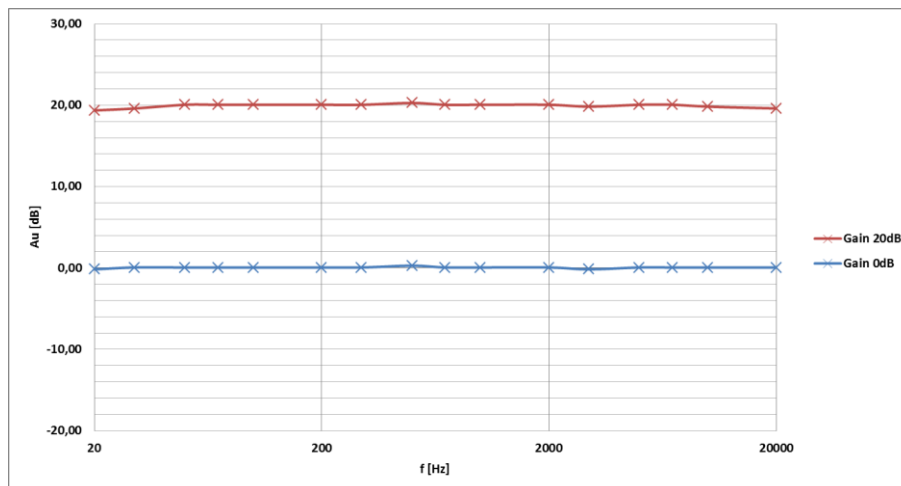
Obr. 4.9: Modulová frekvenční charakteristika předzesilovače 5./6. (stejný pro oba stereo kanály).
