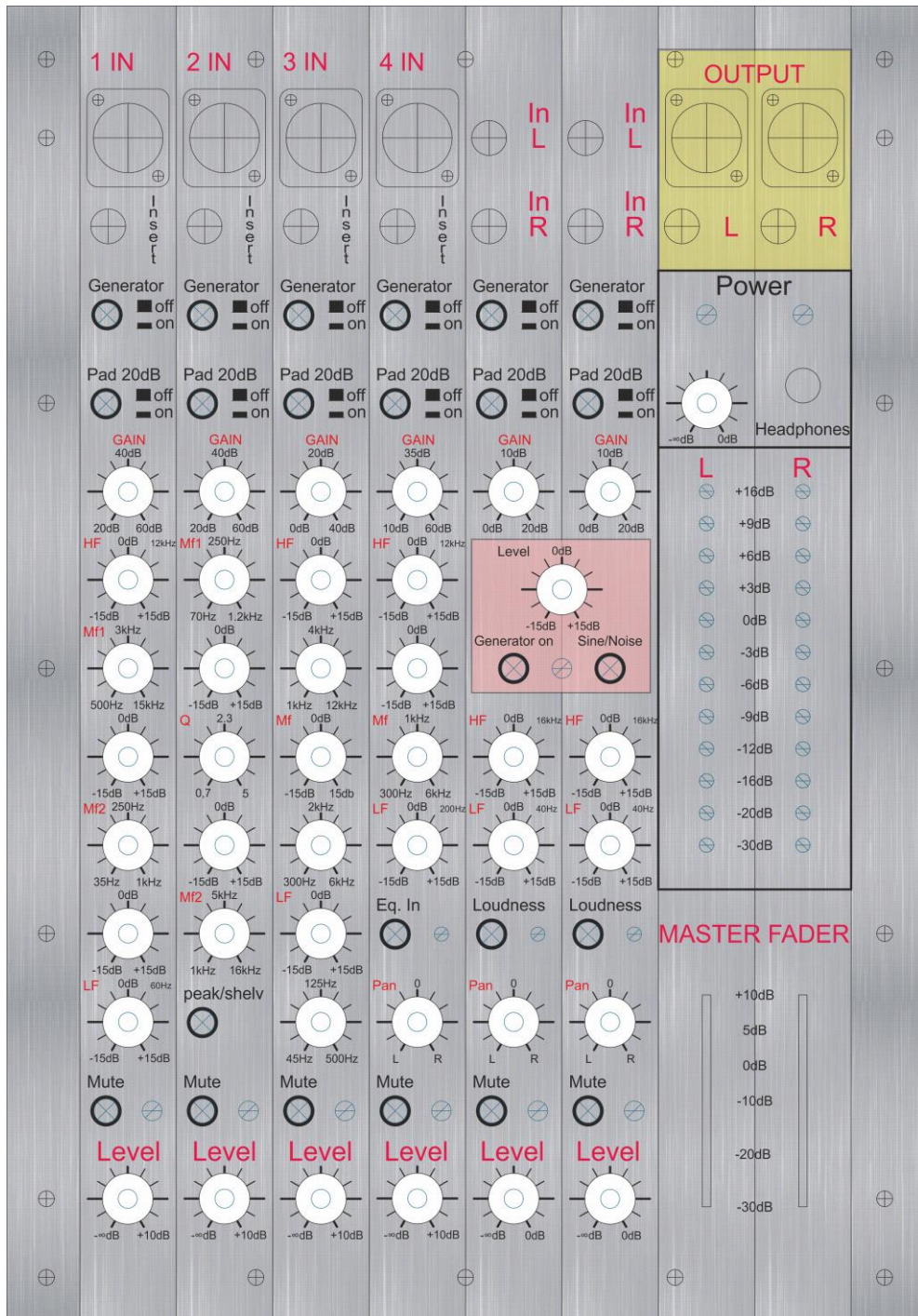
Obr. 3.6: Ovládací panel.
