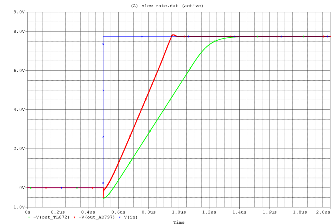
Obr. 2.1: Rychlost přeběhu.
