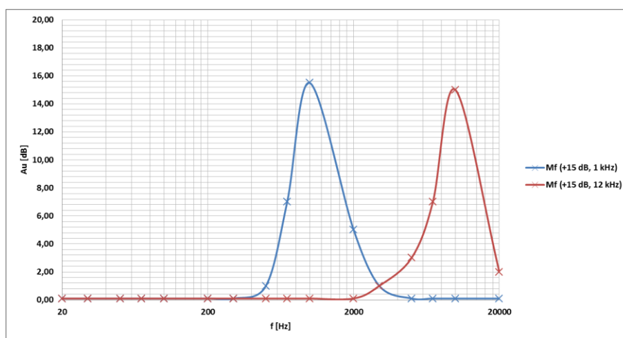
Obr. 4.6: Modulová frekvenční charakteristika ekvalizéru, 3. kanál.
