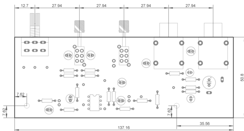
Obr. 3.2: Rozměry DPS pro stereo předzesilovače.
