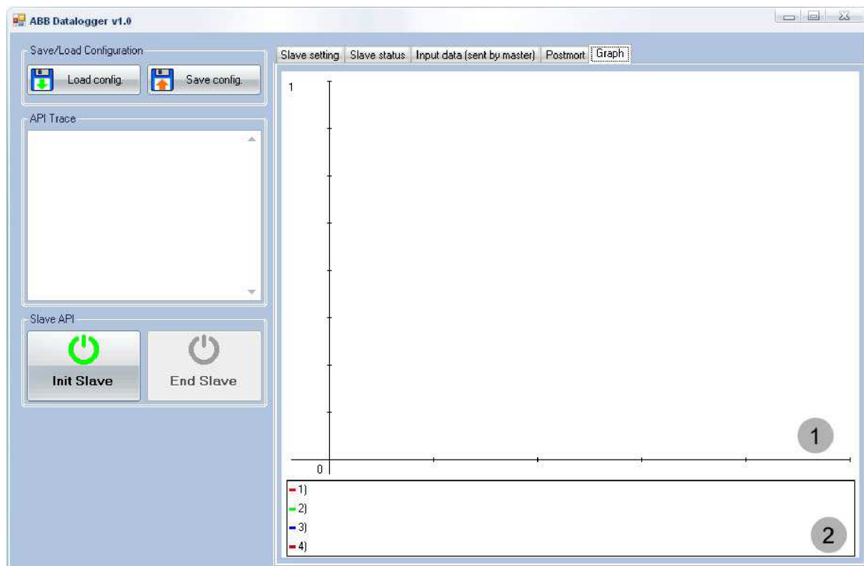
Obr. 23 Zálůžka „Graph“
