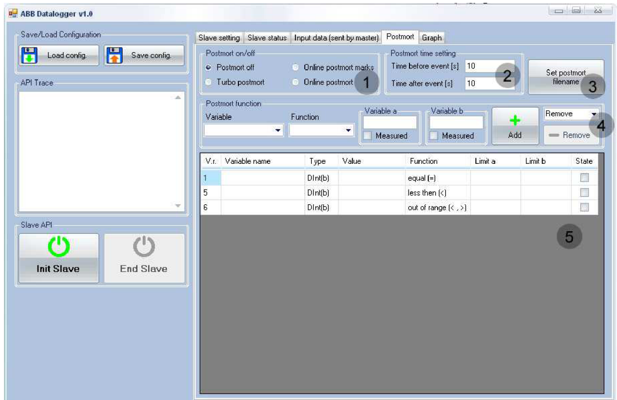
Obr. 22 Záložka „Postmort“
