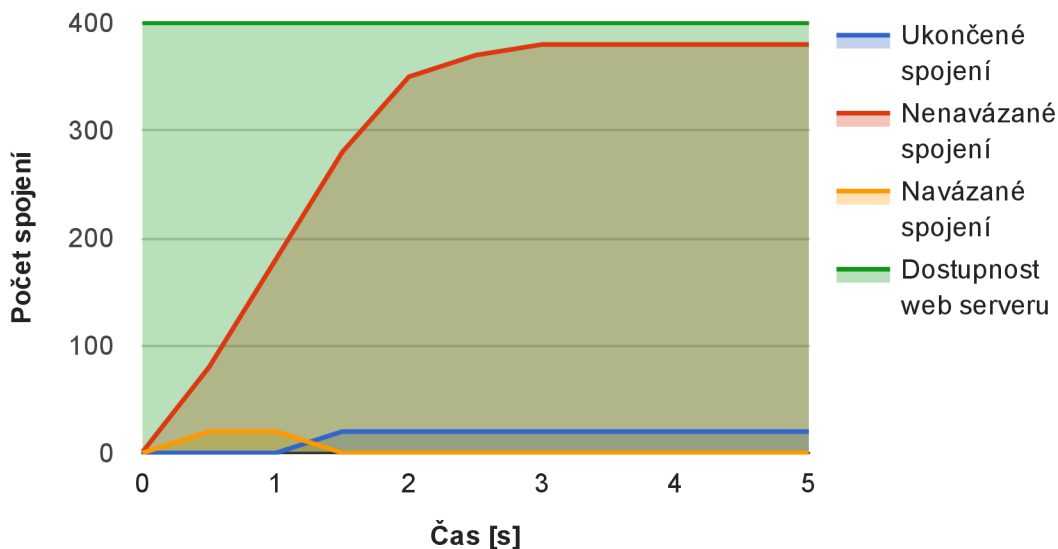
Obr. 6.3: Průběh útoku Slow GET s IPS
