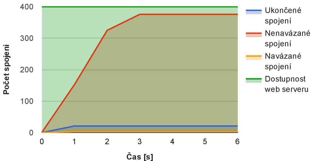
Obr. 6.7: Průběh útoku Range Header s IPS
