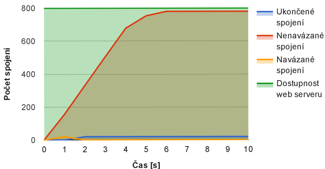
Obr. 6.9: Průběh útoku Slow Read s IPS
