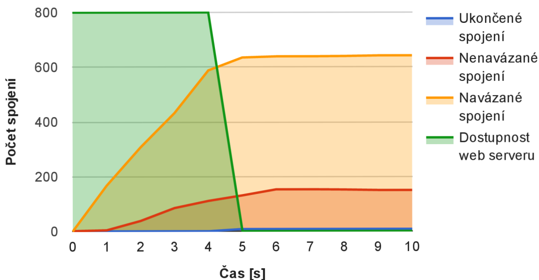
Obr. 6.8: Průběh útoku Slow Read bez IPS
