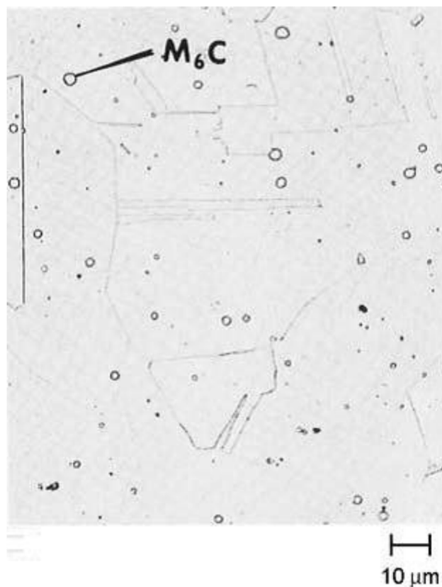
Obr. 8: Mikrostruktura slitiny HAYNESS 188 v žíhaném stavu [14]
