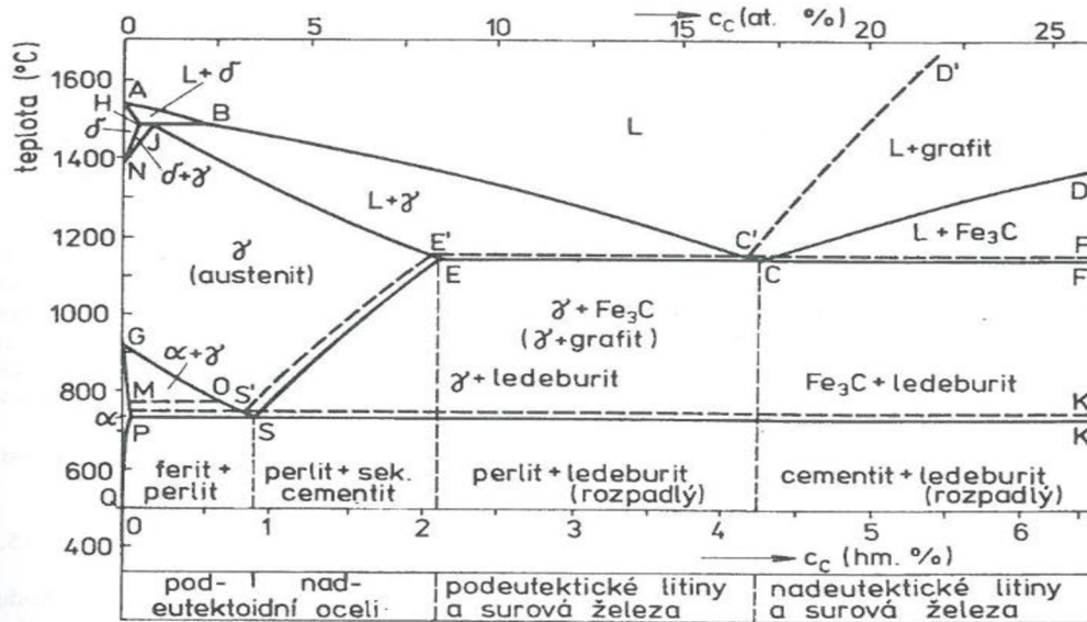
Obr. 4: Rovnovážný diagram soustavy železo – uhlík [5]
