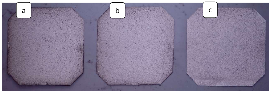
Obr. č. 41 - Omítka D250 - 1 po procesu umělého špinění a) elektrostatický vliv b) mechanický vliv c) vliv termoprecipitace
