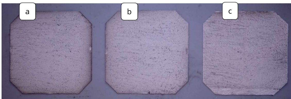
Obr. č. 45 - Omítka F1S - 1 po procesu umělého špinění a) elektrostatický vliv b) mechanický vliv c) vliv termoprecipitace
