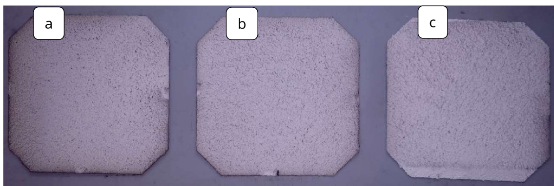
Obr. č. 40 - Omítka D15 - 1 po procesu umělého špinění a) elektrostatický vliv b) mechanický vliv c) vliv termoprecipitace
