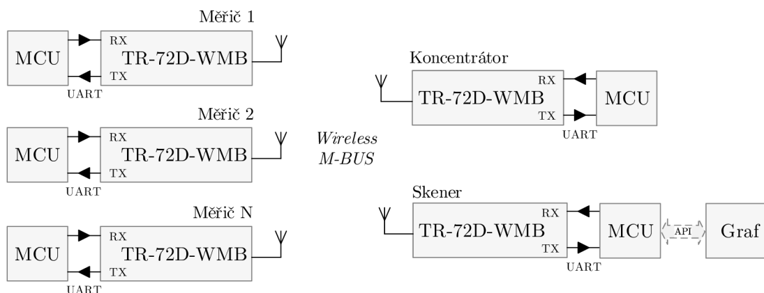
Obr. 4.4: Různé módy dle použité topologie [46]
