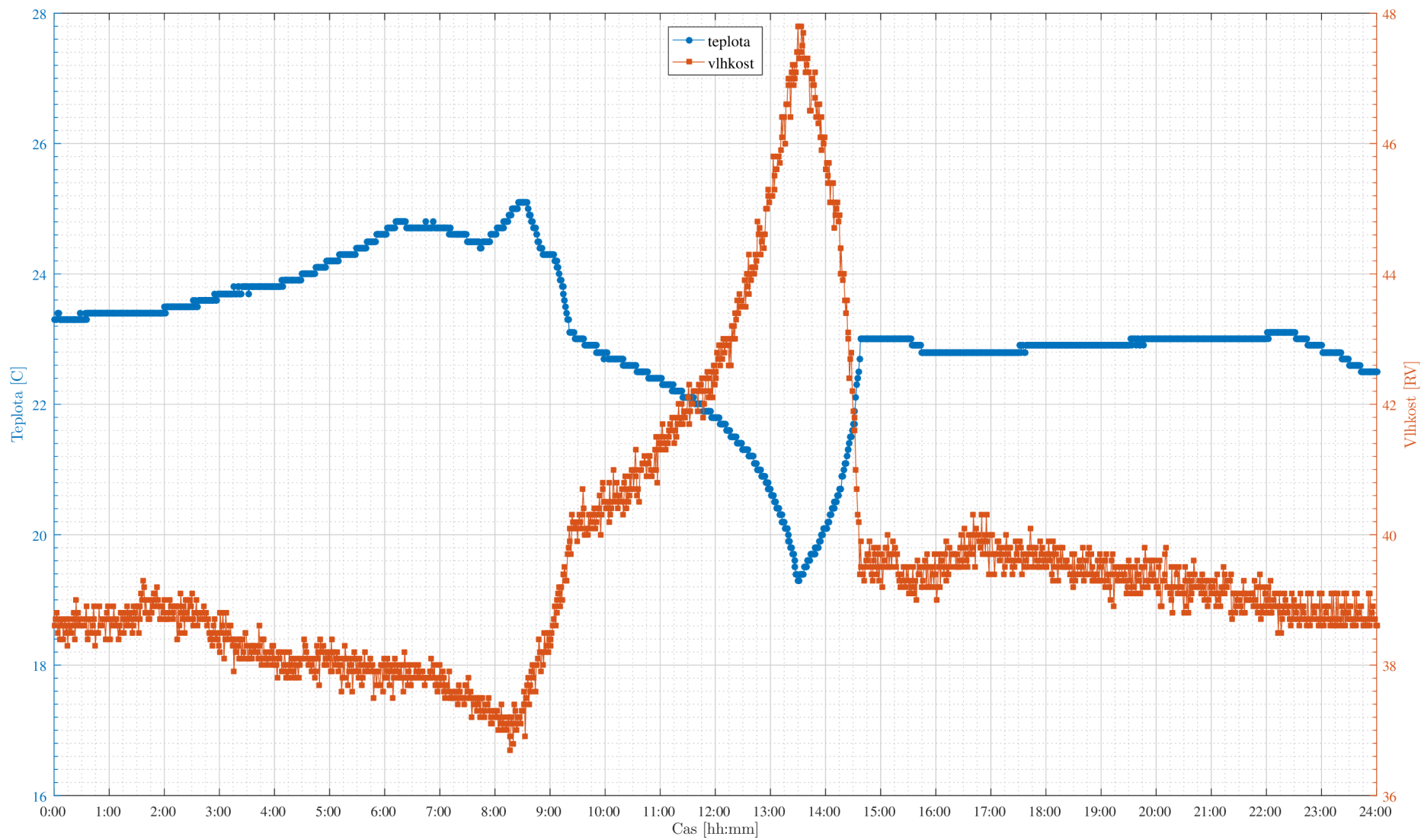
Obr. C.3: Vizualizace měření čidlem Weptech (interval 24 hodin)
