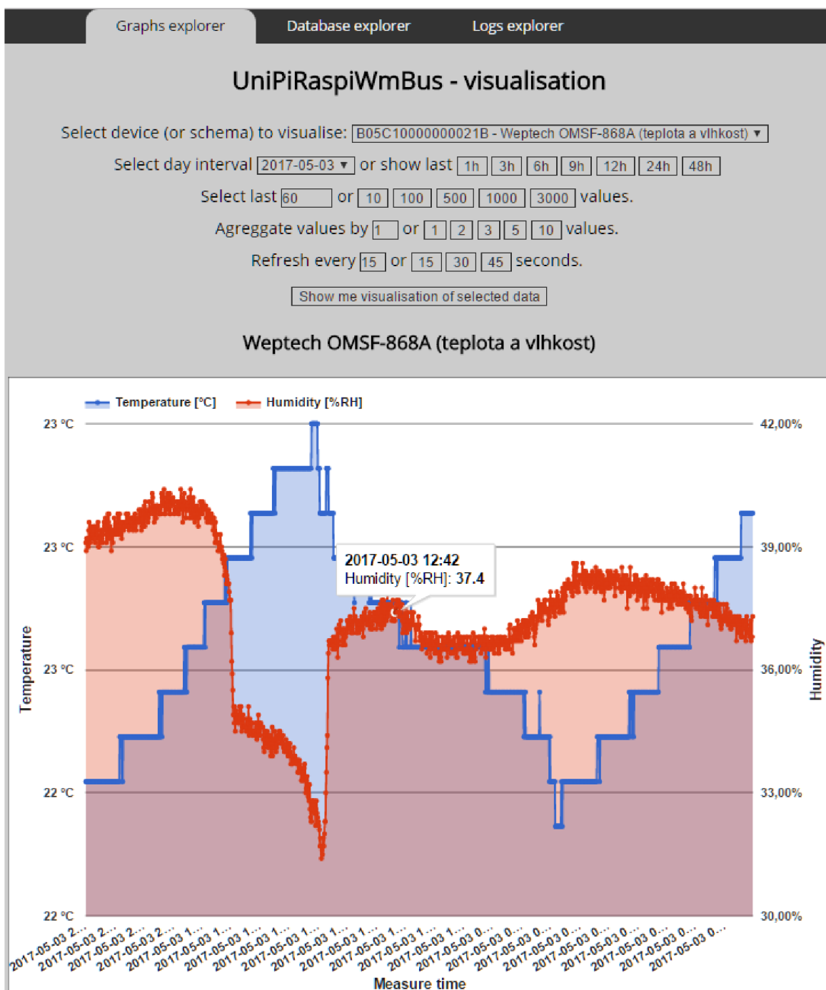
Obr. 7.3: Snímek obrazovky vizualizační aplikace
