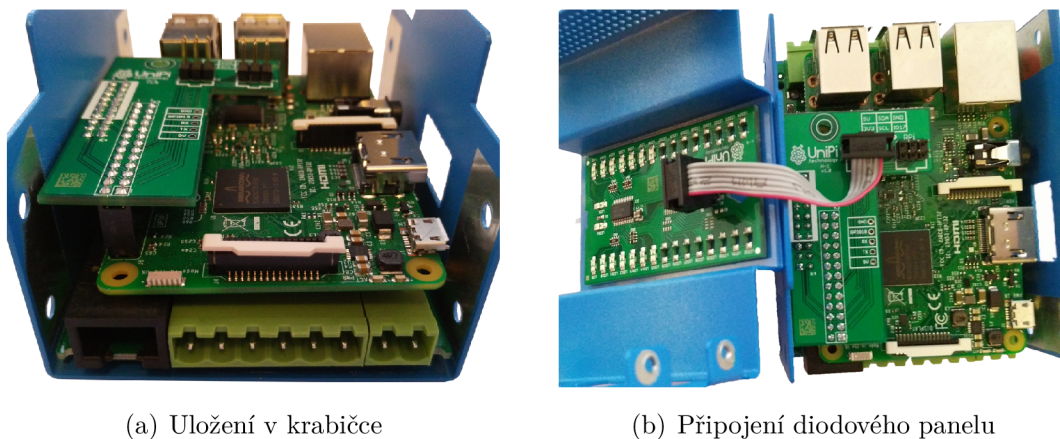
Obr. 3.6: Detaily vnitřního uspořádání UniPi Neuronu S103
