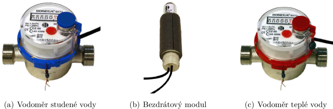
Obr. 6.2: Sada Bonega [60]
