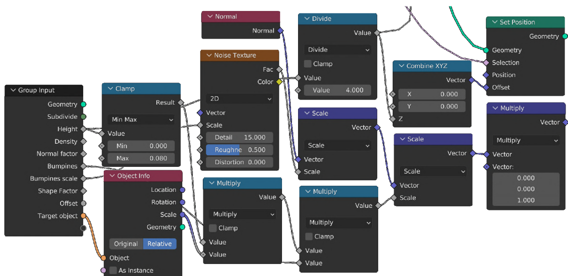
Obr. 4.4: Strom uzlov pridávajúci vygenerovanému snehu hrboľatosť pomocou noise textúry a modifikujúci výšku objektu. Z postupnosti uzlov je vidno že nieje možné použiť vytiahnutie geoemtrie na kontrolu výšky, ale je potrbné modifikovať pozíciu v Z-ovej osi pre vrchné plochy vytiahnutej geoemtrie. Taktiež je vidieť že veľkosť textúry šumu je násobená veľkosťou objektu, aby v prípade nejdenotnej veľkosti objektu, vygenerovaný sneh, zachoval veľkosť hrboľov
