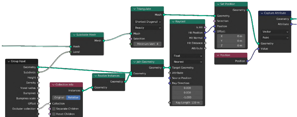
Obr. 4.9: Strom uzlov, ktorý vykonáva raycast a zachytáva pozíciu dopadnutých lúčov. Geometrie plochy je najskôr potrebné rozdeliť, aby sme mali viac detailov pre generovanie snehu.
