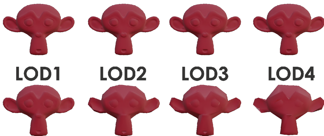
Obr. B.1: Nástroj na generovanie levelu detailov pre objekty. Je možné vidieť že každá úroveň postupne znižuje na definíciu geometrie.
