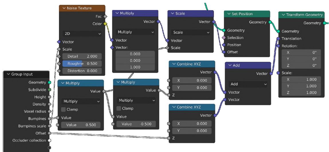
Obr. 4.12: Strom uzlov, ktorý pridáva snehu hrboľatosť a posúva ho v osi Z. Pre pridanie hrboľatosťi je použitá textúra šumu, ktorej veľkosť je násobená veľkosťou objektu, aby sa zachovali veľkosti hrboľov aj pri nerovnomernej veľkosti objektu.
