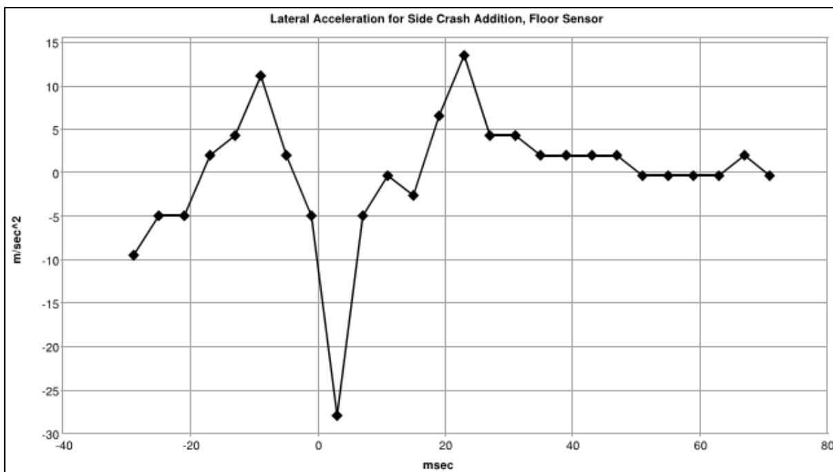
Obr. č. 28 – Graf bočního zrychlení vozidla (snímač na podlaze vozidla) [52]
