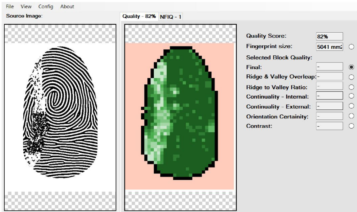
Obr. 6.8: Vyhodnotenie jazvy s čiernymi útvarmi aplikáciou FiQiVi vrátane mapy kvality. Pôvodný problém s určením jazvy ako pozadia sa pridaním čiernych útvarov eliminoval.
