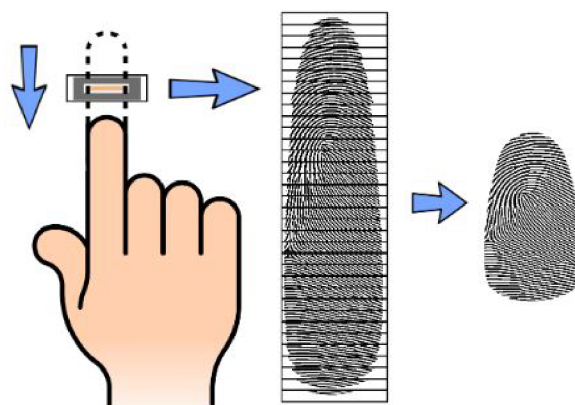
Obr. 3.2: Princíp fungovania prietahového snímača. Prevzaté z: [27].
