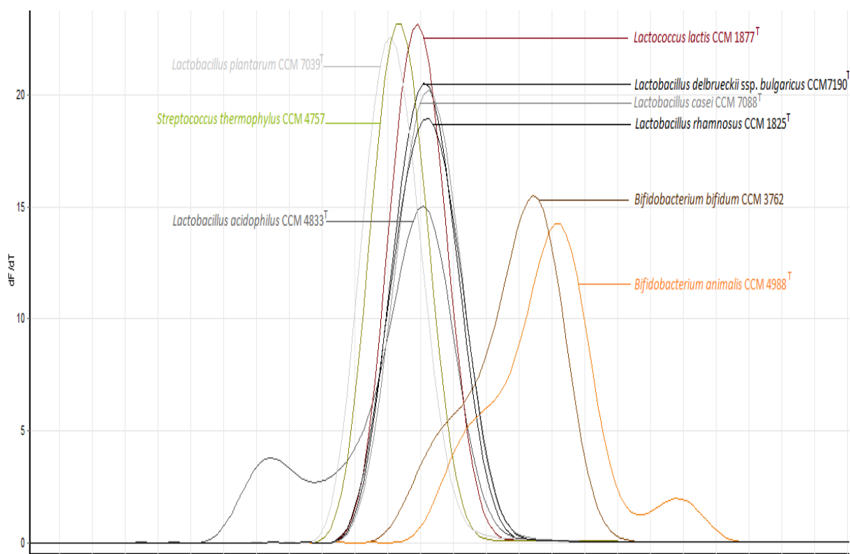
Obrázek 19: Křivky tání DNA kmenů použitých jako pozitivní kontroly pro RT-PCR s primery V6_F, V6_R
