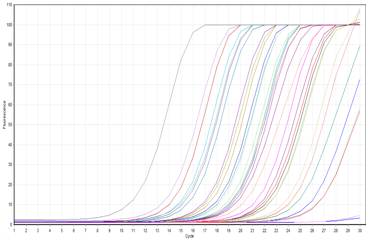
Obrázek 8: Amplifikační křivky RT-PCR s primery specifickými pro doménu Bacteria
