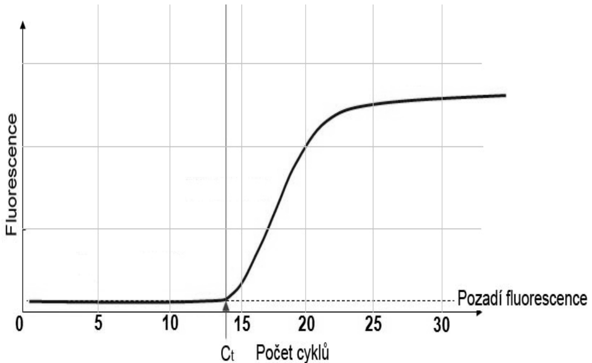
Obrázek 5: Amplifikační křivka, upraveno podle [27]
