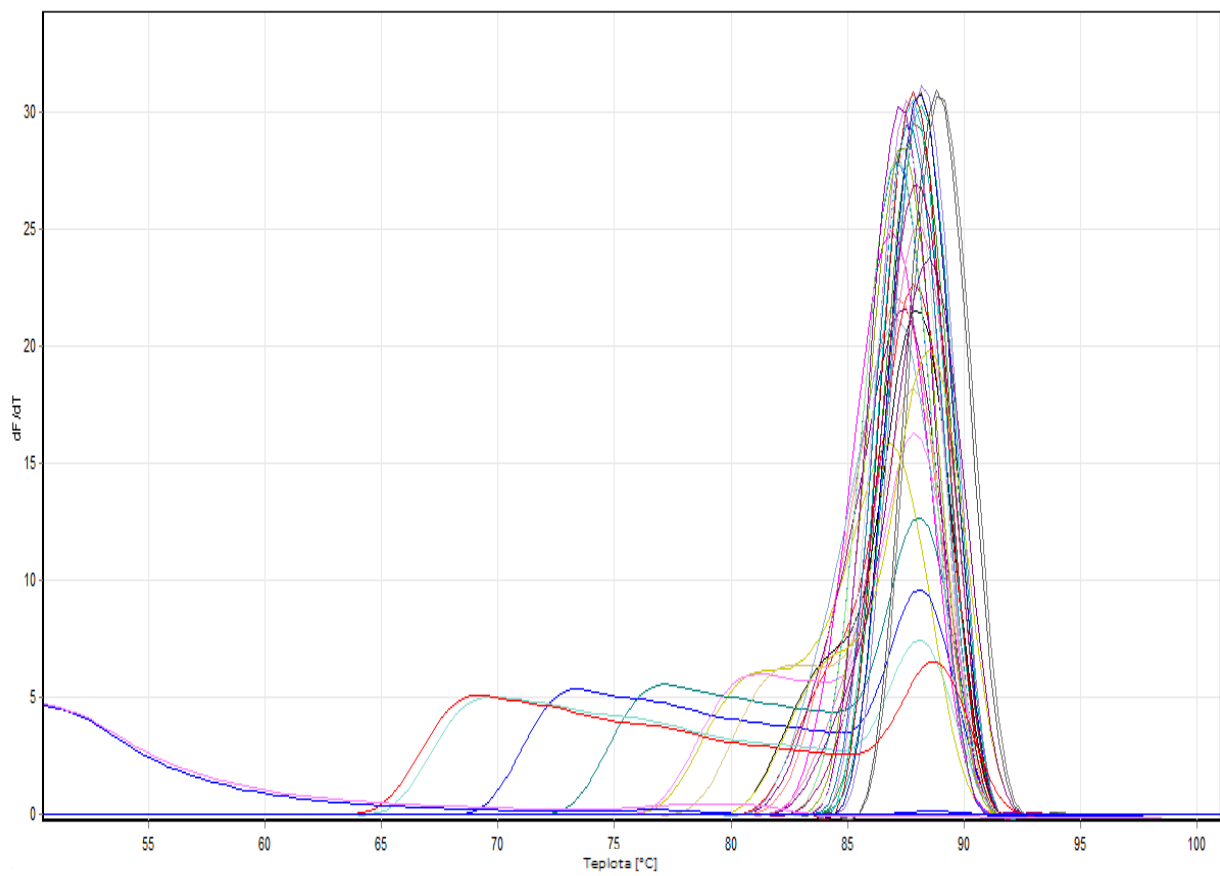
Obrázek 9: Analýza křivek tání produktů RT-PCR s primery specifickými pro doménu Bacteria
