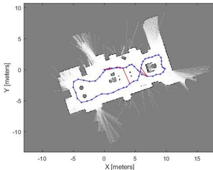
Obr. 1.6 Virtuální mapa vytvořená technologií LiDAR SLAM
