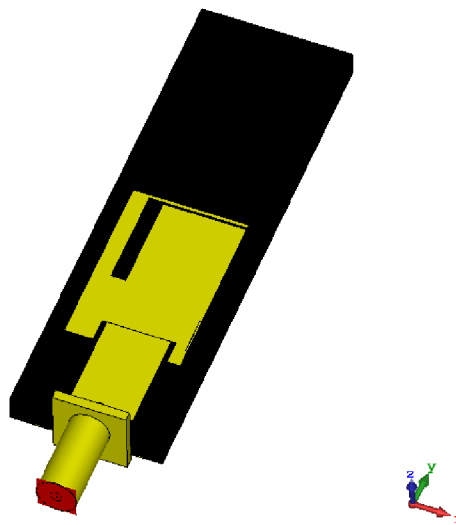
Obrázek 4.4 PIFA verze 1 s přechodem konektor - mikropásek
