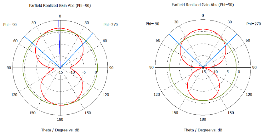
Obrázek 3.6 Zisk PIFA při 1,8 GHz (levý obrázek) při 2,4 GHz (pravý obrázek) v rovině YZ.
