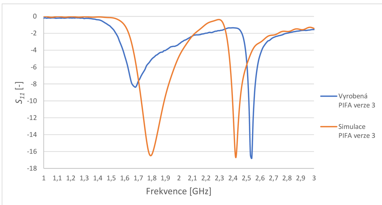
Obrázek 5.6 Činitel odrazu vyrobené PIFA verze 3 umístěné na PLA oproti simulaci této verze
