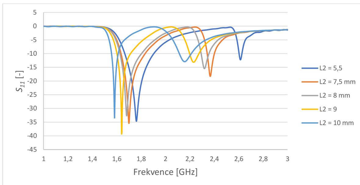
Obrázek 4.17 Činitel odrazu PIFA, při rozmitání parametru L2
