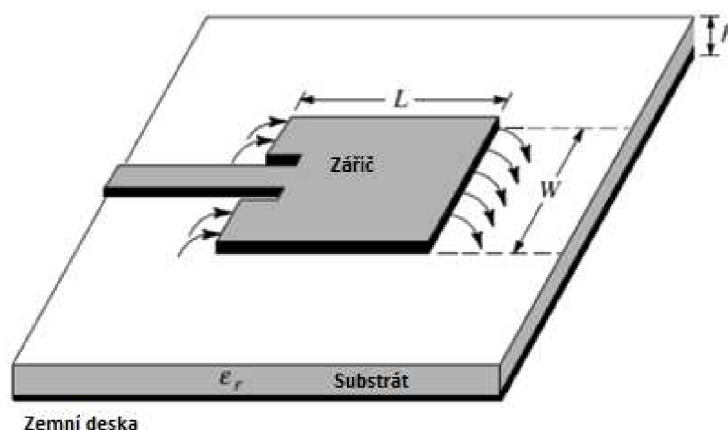
Obrázek 1.1 Jednopásmová patch anténa napájena mikropáskem [3].
