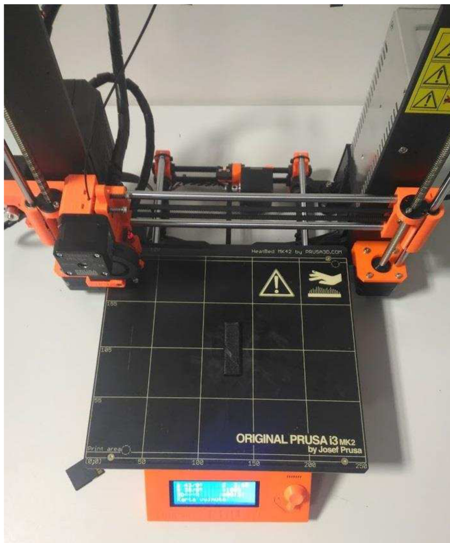
Obrázek 5.1 Ukázka 3D tiskárny ORIGINAL prusa i3 MK3 společně s vytištěným dielektrikem z PLA
