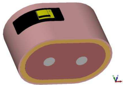
Obrázek 3.12 Oválný model lidské ruky s větší vrstvou svalu společně s PIFA
