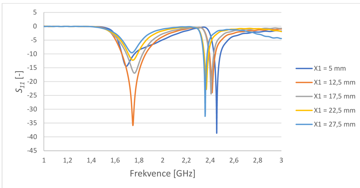
Obrázek 4.19 Činitel odrazu PIFA, při rozmitání parametru X1
