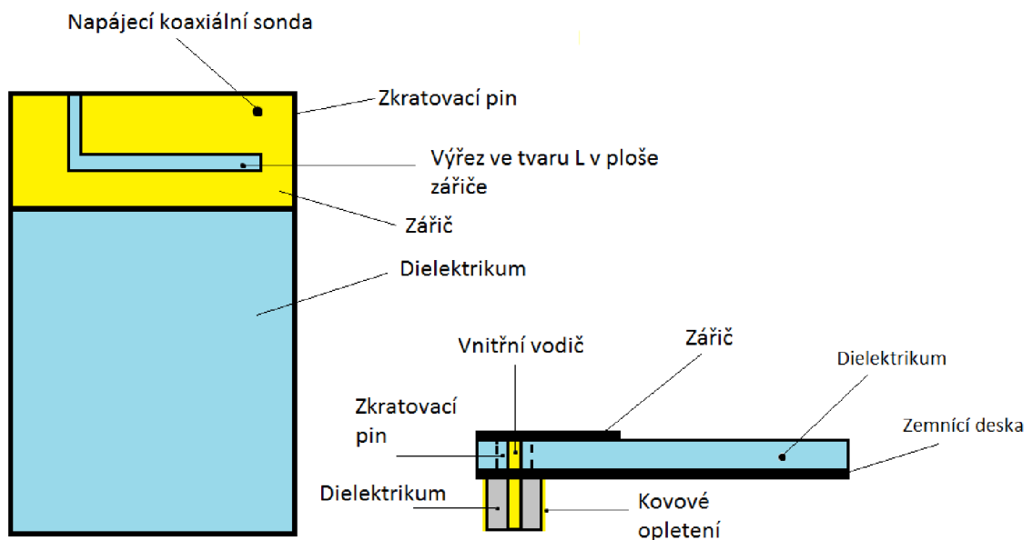
Obrázek 2.4 Ukázkou dvoupásmové PIFA.
