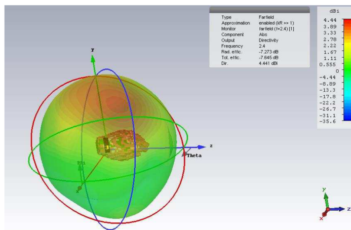
Obrázek 3.19 Směrovost PIFA umístěné na voxelovém modelu lidské ruky při 2.4 GHz.
