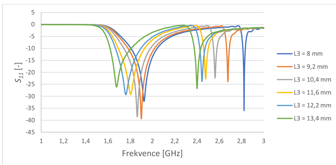
Obrázek 4.18 Činitel odrazu PIFA, při rozmitání parametru L3
