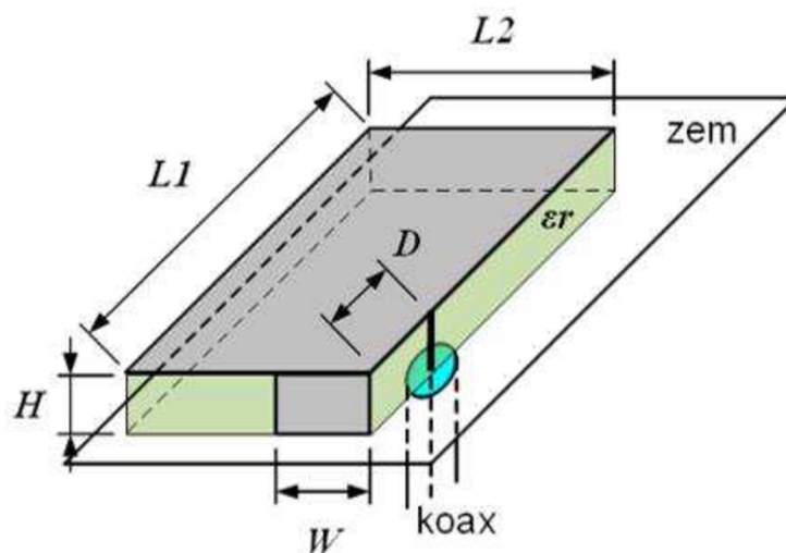
Obrázek 2.1 PIFA[5]
