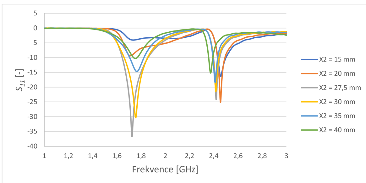
Obrázek 4.20 Činitel odrazu PIFA, při rozmitání parametru X2
