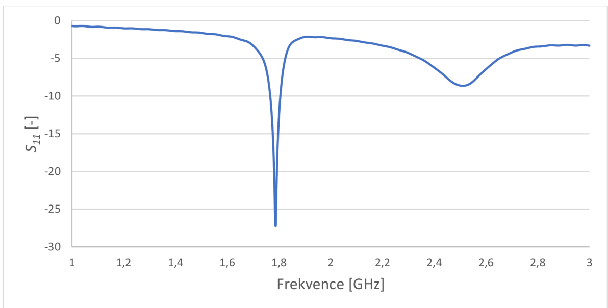
Obrázek 3.15 Činitel odrazu pro oválný model lidské ruky na obrázku 5.14.
