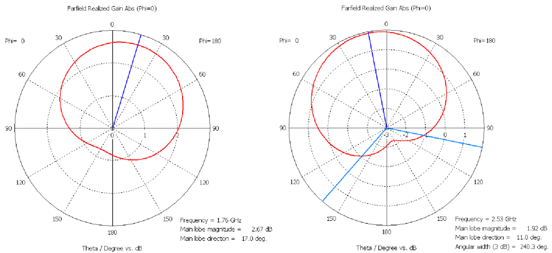
Obrázek 4.13 Zisk PIFA verze 3 v rovině H, tedy XZ pro oba kmitočty (1,76 GHz vlevo a 2,53 GHz vpravo)
