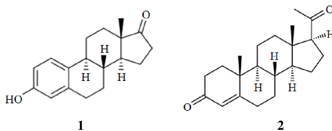
Obr. 3. Struktura estrogenu (1) a progesteronu (2).
