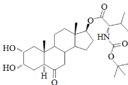
Obr. 13. Struktura původní účinné látky bez linkeru pro navázání, MK-349 [(2 \alpha ,3 \alpha -dihydroxy-6-oxo-5 \alpha -androstan-17 \beta -yl)-N-( tert -butoxykarbonyl)-L-valinát].
