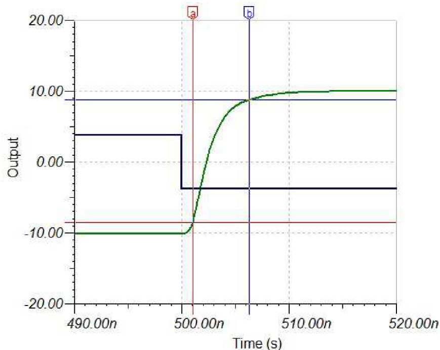
Obr. 2.8: Simulovaná rýchlosť priebehu zapojenia pri rozkmit výtupu 20\text{V}_{pp}/50\Omega
