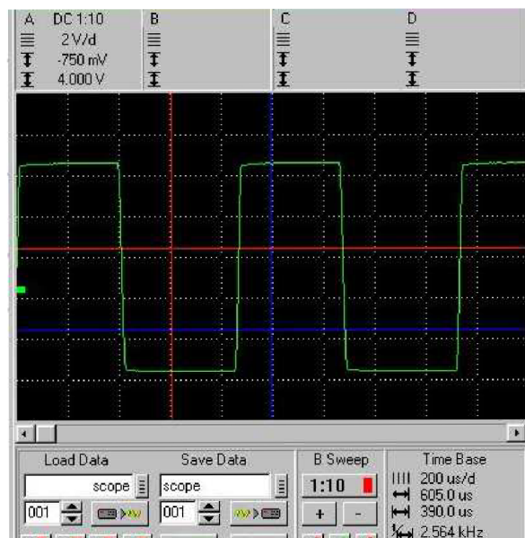
Obr. 3.3: Obdĺžnikový priebeh 10 Vpp pri zát'aži 50 Ω, 1,14 kHz
