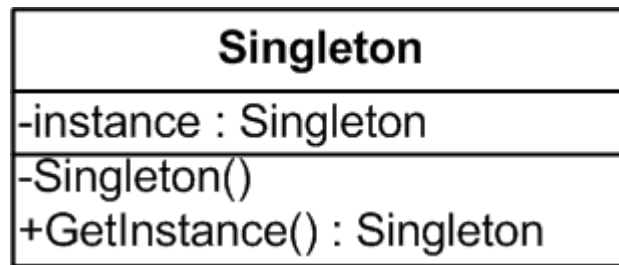
Obr. 2 - UML diagram
