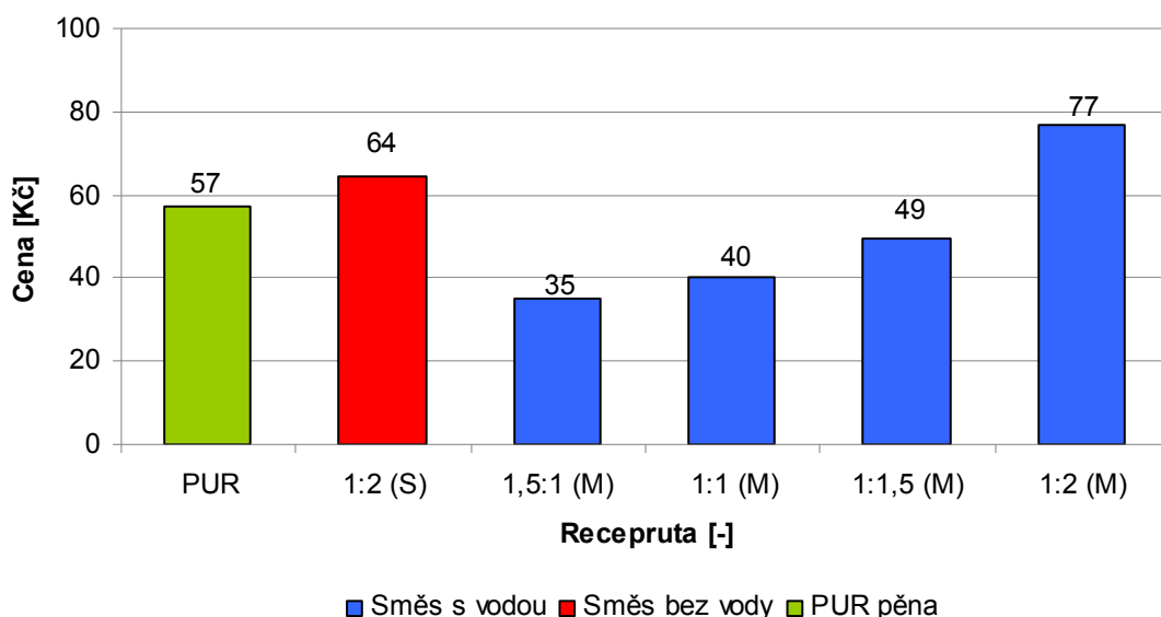
Graf 20: Porovnání ceny integrované izolace v keramické zdičce tvarovce PTH 30 T.
