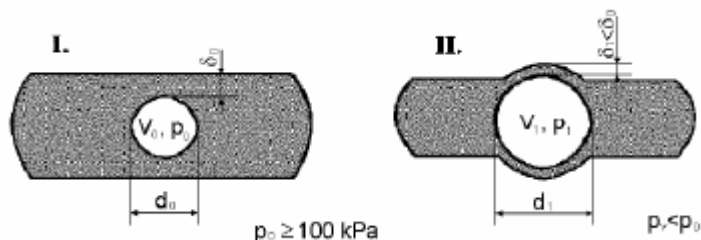
Obr. 3: Princip vakuování, I. Velikost póru při atmosférickém tlaku, II. vakuováním dochází ke snížení okolního tlaku, čím se zvětší vzduchový pór až do jeho prasknutí/odstranění [11].
