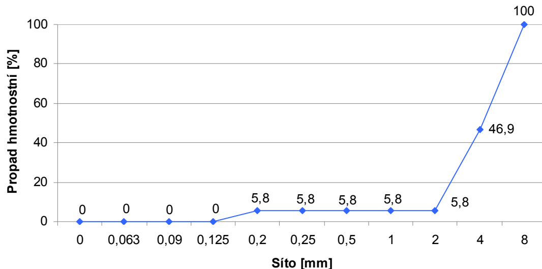
Graf 7: Křivka zrnitosti PUR 3-5.
