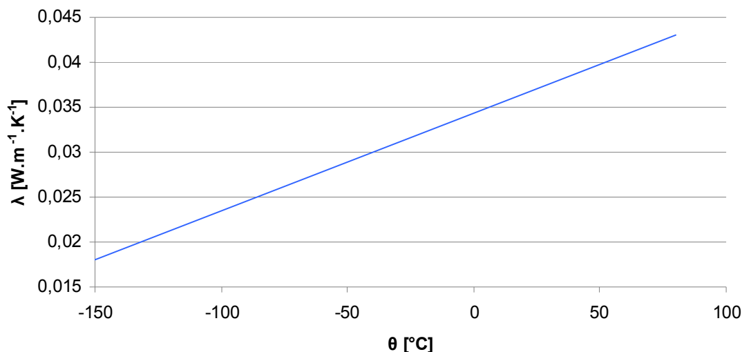
Graf 6: Vliv teploty na součinitel tepelné vodivosti EPS. Měřeno na vzorku s objemovou hmotností 20 \text{ kg.m}^{-3} [19].
