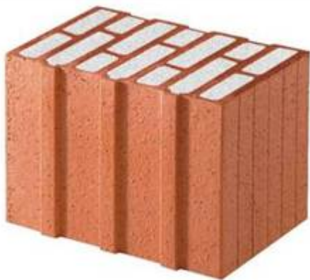
Obr. 26: Keramická zdící tvarovka Poroton T [29].
