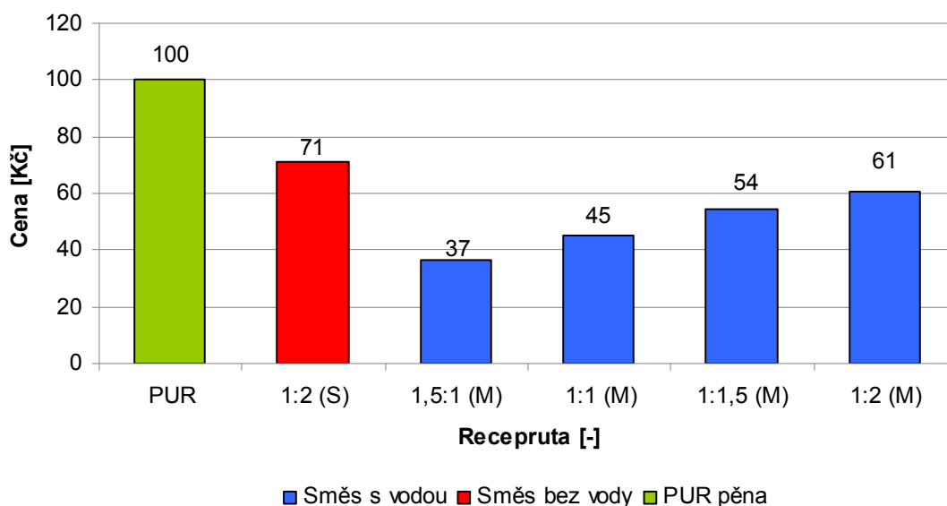
Graf 18: Porovnání ceny za 1 \text{ m}^3 jednotlivých integrovaných izolantů.
